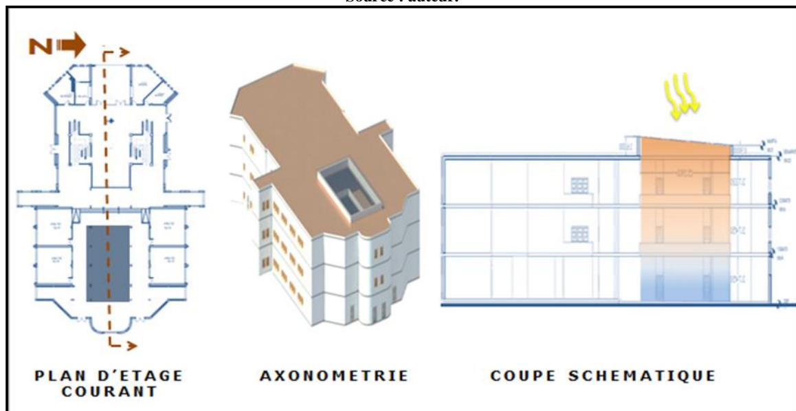
Figure II. 21 : Modélisation du bâtiment des sciences islamiques.
