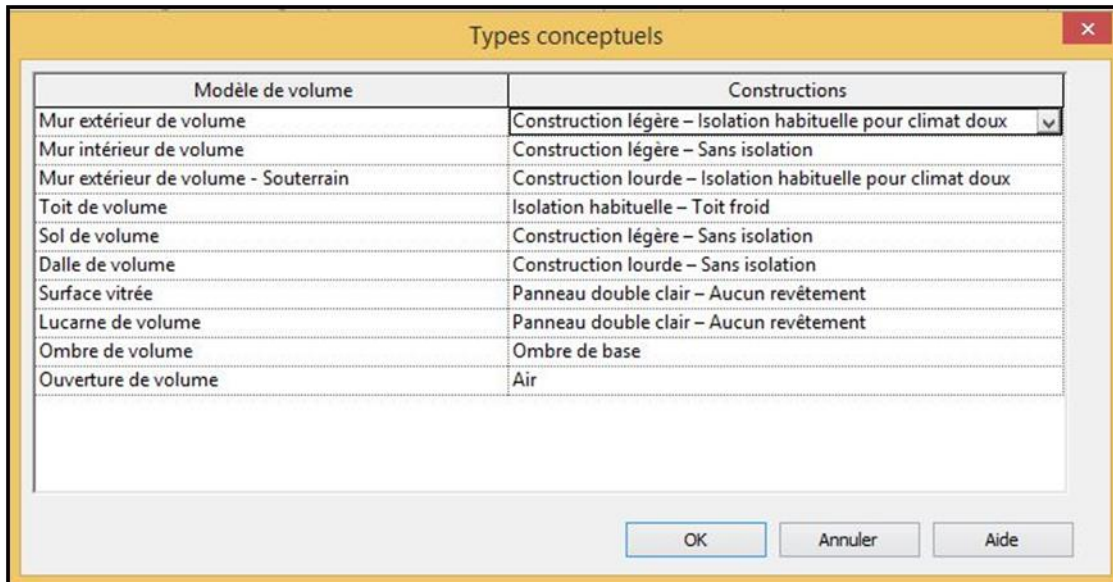
Figure V. 46 : les éléments constructifs dans logiciel. Source : auteur.
