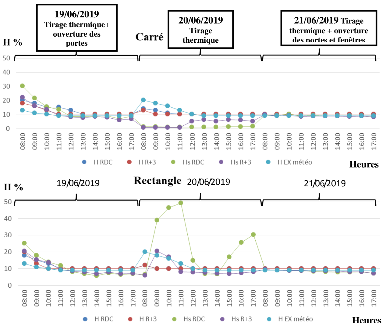
Figure IV. 36 : L'humidité relative de l'air (R+3 Polycarbonate).
