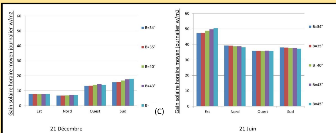
Figure IV. 5 : Taux d'irradiation solaire en solstices d'hiver et d'été selon les quatre orientations. Source : Auteur.
