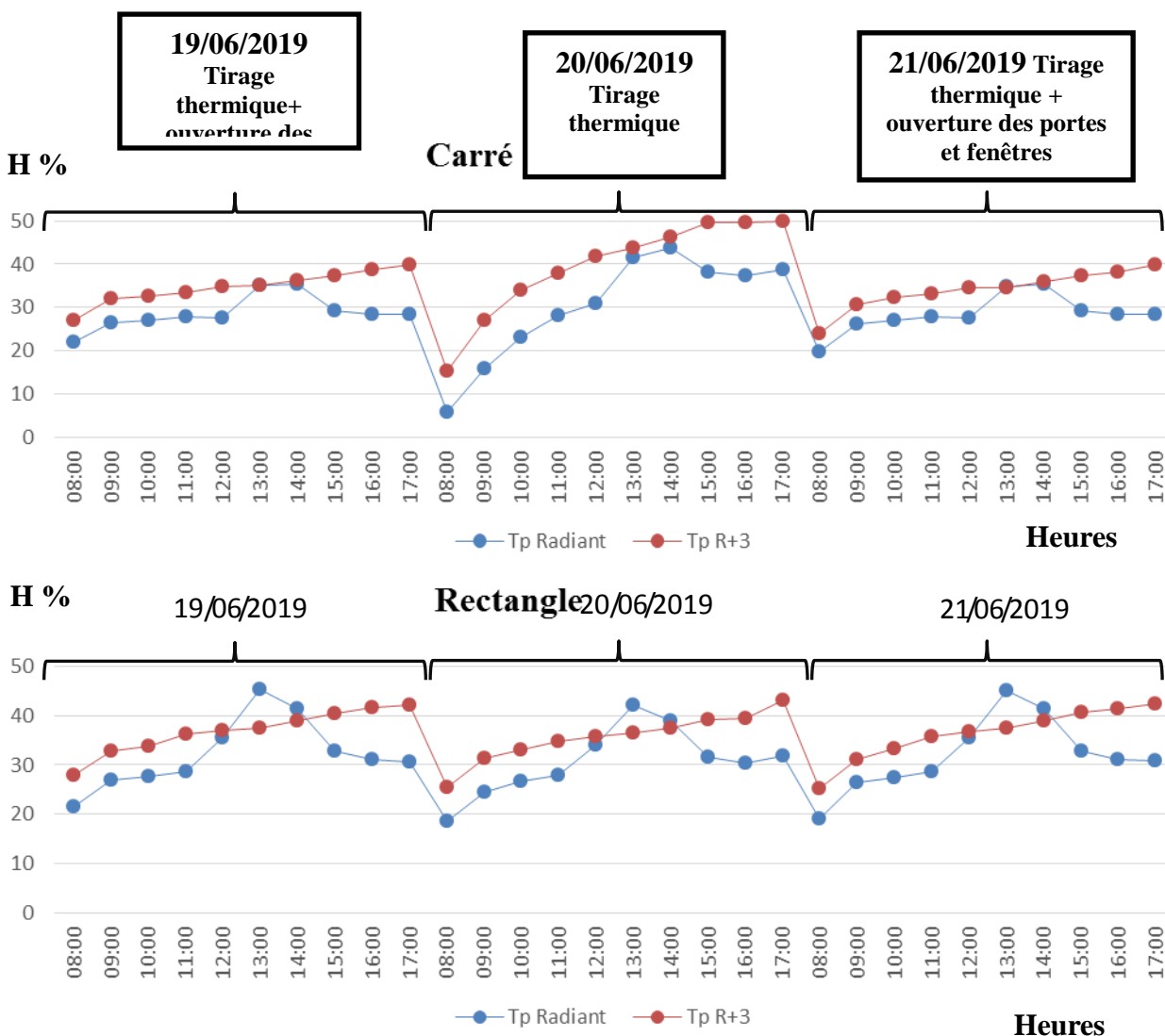
Figure IV. 37 : La température radiative moyenne (R+3 Polycarbonate). Source : auteur.
