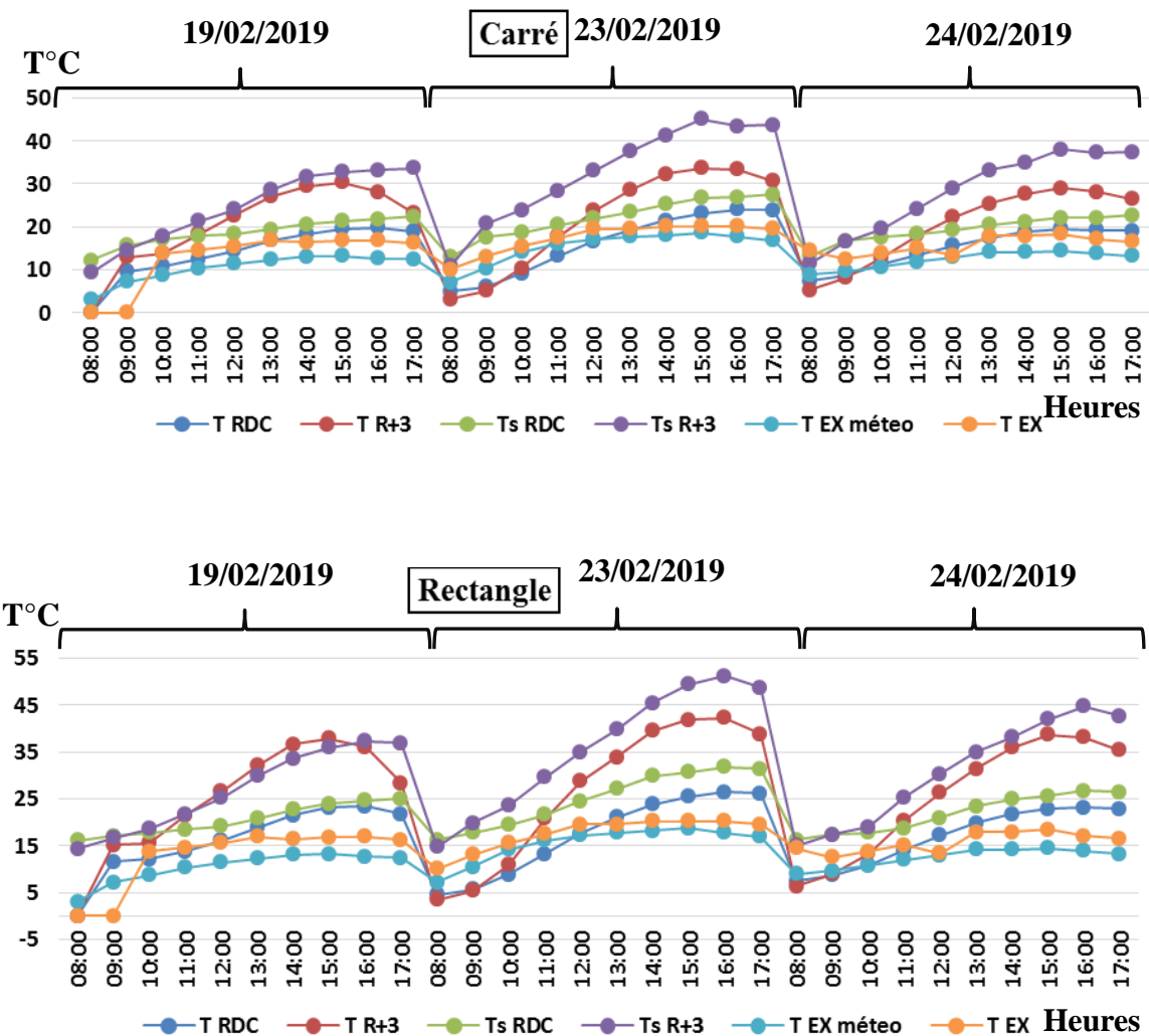
Figure IV. 15 : La température de l'air (R+3 Double vitrage) carré et rectangle.
