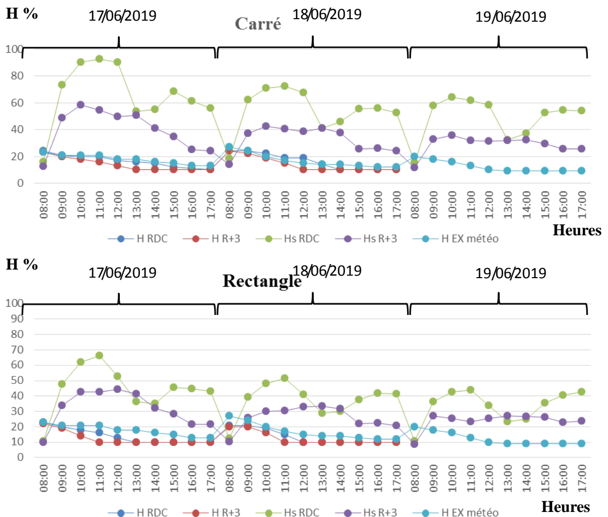
Figure IV. 32 : L'humidité relative de l'air (R+3 Polycarbonate). Source : auteur
