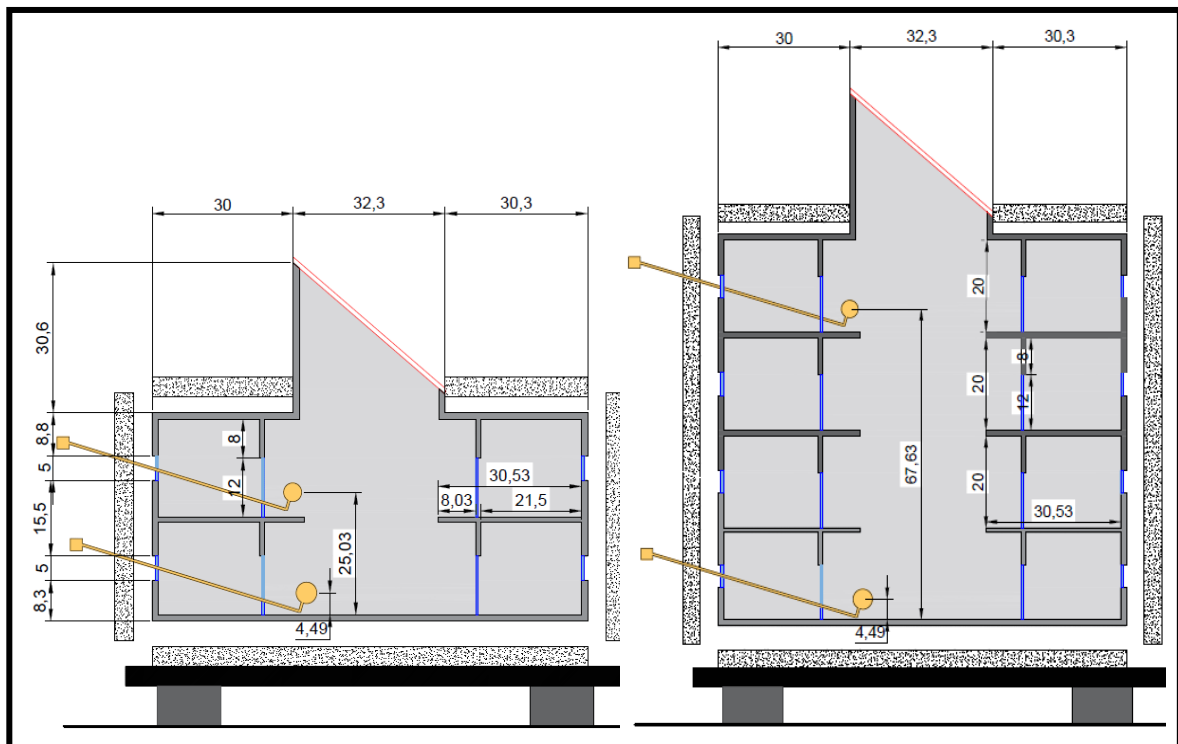
Figure IV. 13 : Coupe schématique sur les maquettes.
