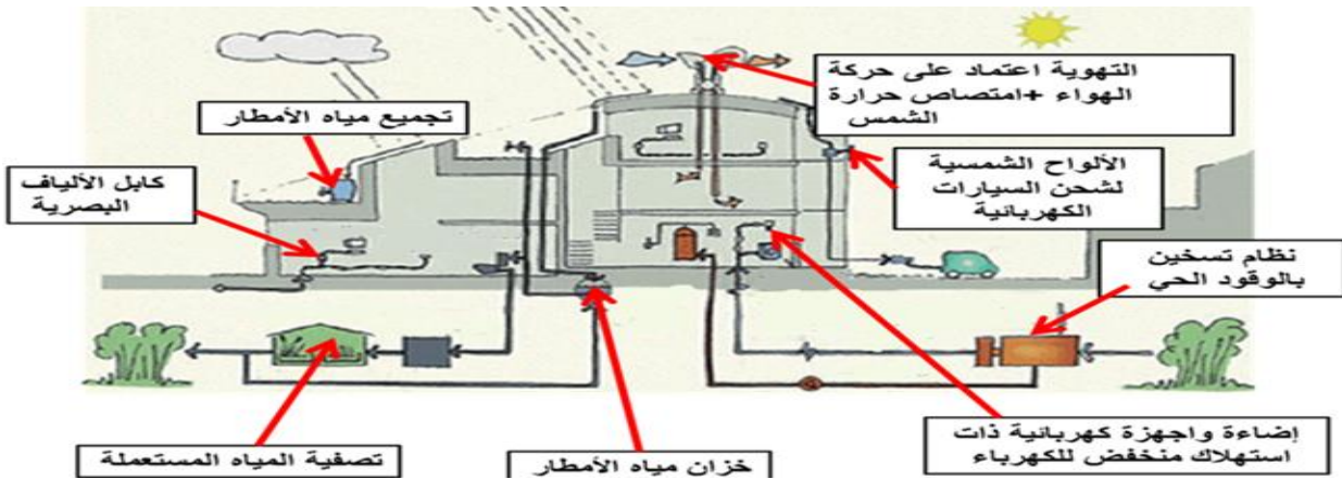
الصورة رقم (33) – توضح مخطط التهوية والتدفئة ودورة تخزين واستعمال مياه الأمطار والدارة الكهربائية في إحدى المساكن المصدر: بحث حول الحي الايكولوجي من إعداد الطلبة بوزارة نسرين و بوعبيدي إيمان و بوعيشة سليمة الفوج 1. 2015/2014.
