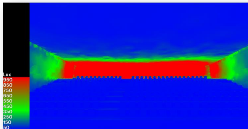
Figure VI 23: Niveau d'éclaircement en false colour. Source : auteur
