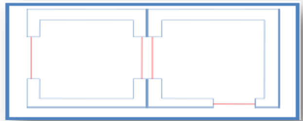
Figure VI 3: ouvertures latéral parallèles et perpendiculaires pour un éclairage bilatéral (source : auteur).
