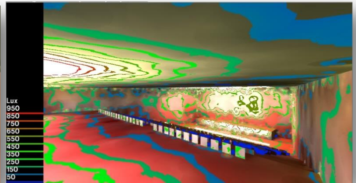
Figure VI 29: Niveau d'éclairage en contour bands. Source : auteur
