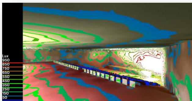
Figure VI 28: Niveau d'éclairage en contour bands. Source : auteur
