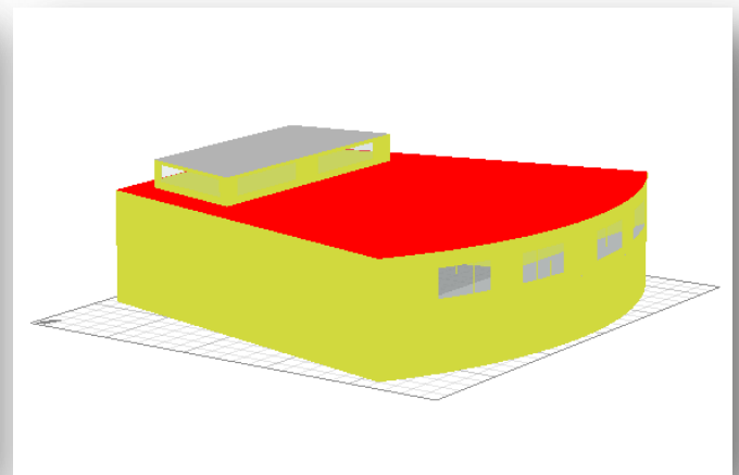
Figure VI 26: vue de la toiture ( éclairage zénithal.) Source : auteur
