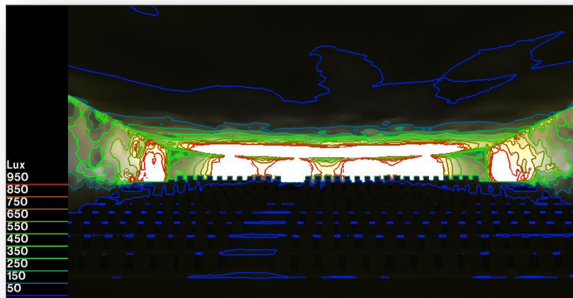
Figure VI 18: Niveau d'éclairage en contour lignes source : auteur
