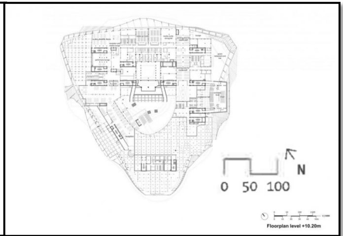
Figure I.23 : plan de 1 er étage. Source : http://www.coop-himmelblau.at
