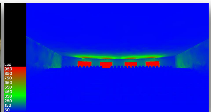
Figure VI 20: Niveau d'éclairage en false colour. Source : auteur
