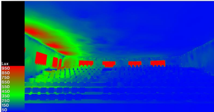
Figure VI 16: Niveau d'éclaircement en fausse couleur. Source : auteur
