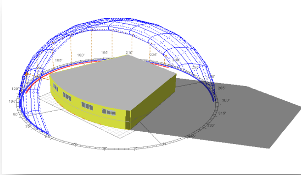
Figure VI 14: l'ombre portée du projet le 22 décembre à 9 heures Source : auteur
