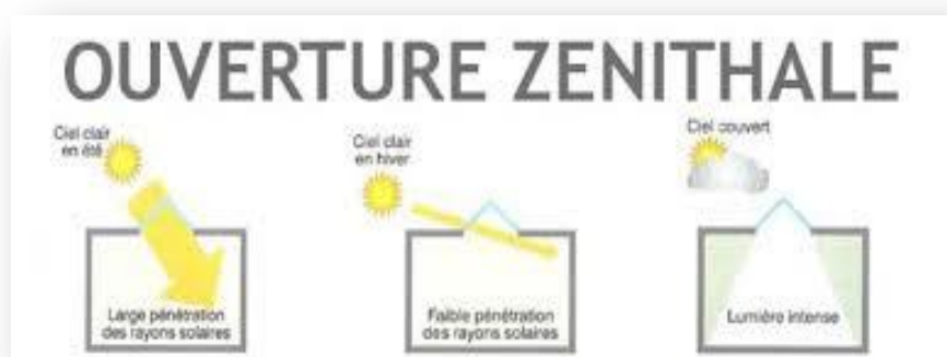
Figure VI 5:les types des ouvertures zénithales Source (A .Liebard et A. De herde, 2005).
