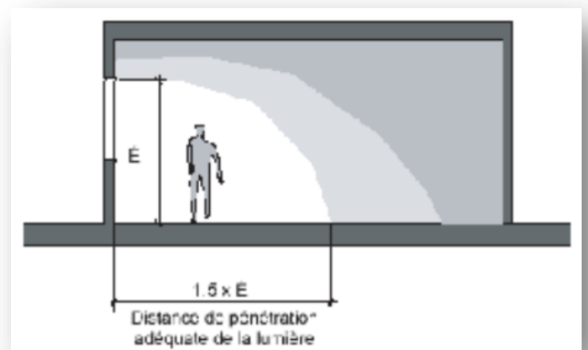
Figure VI 2: pénétration approximative de la lumière naturelle Source : ROBERTSON, Keith. Guide sur l'éclairage naturel des bâtiments
