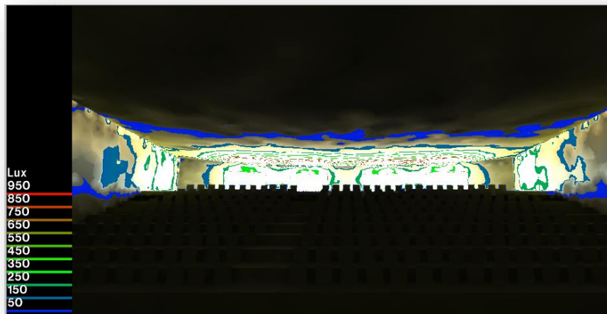
Figure VI 24: Niveau d'éclaircement en contour bands . Source : auteur
