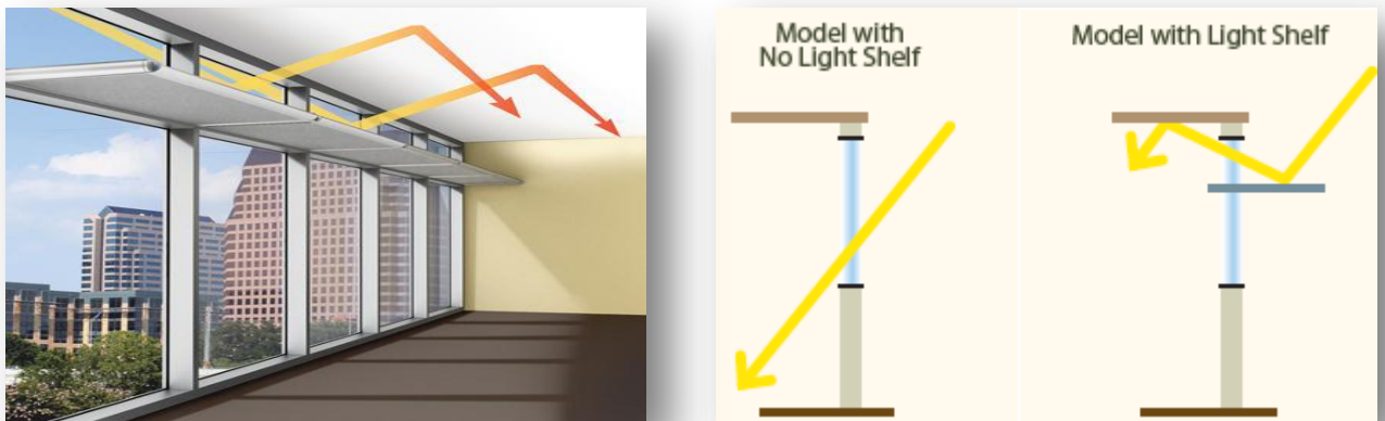
Figure VI 6: fonctionnement d'un lightshelf Source www.energieplus.com
