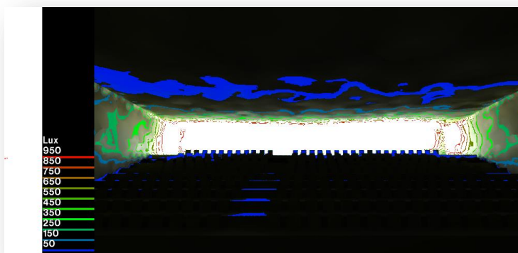
Figure VI 22: Niveau d'éclaircement en contour lines . Source: auteur
