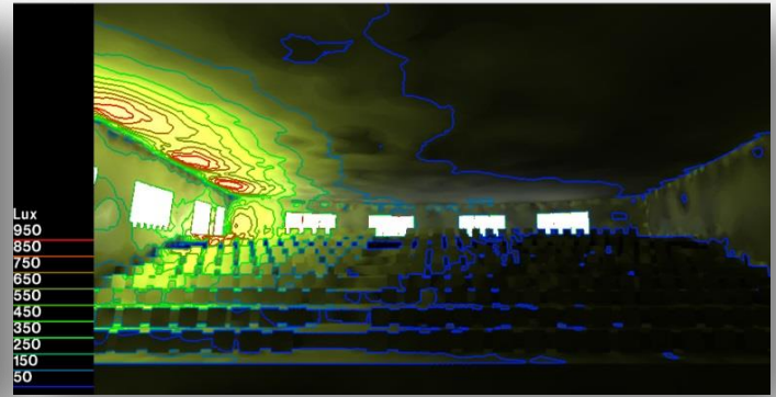
Figure VI 15: Niveau d'éclaircement en contour lignes . Source:auteur
