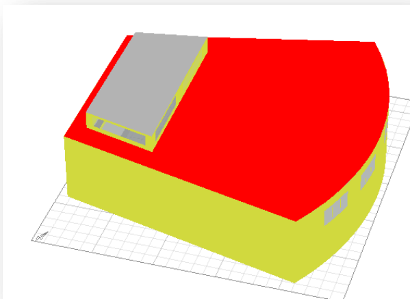
Figure VI 26: vue de la toiture ( éclairage zénithal.) Source : auteur
