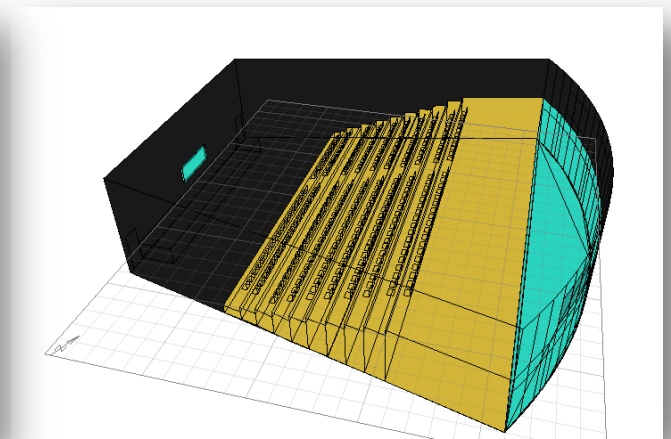
Figure VI 11: vue de l'amphi (cas d'été) Source : auteur
