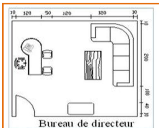
Figure 37: Dimensionnement Source : Neufert 8 ème Edition page 343P
