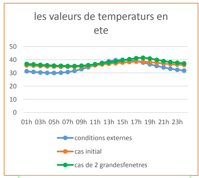
Figure 129: GRAPHE PRESENTE LES VALEURS DE LA TEMPERATURE EN ETE POUR LE CAS AMELIORE N°1
