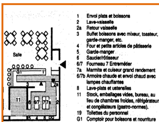
Figure 47: Dimensionnement Source: Neufert 8 ème Edition page 400
