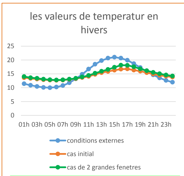
Figure 128: GRAPHE PRESENTE LES VALEURS DE LA TEMPERATURE EN HIVER POUR LE CAS AMELIORE N°1
