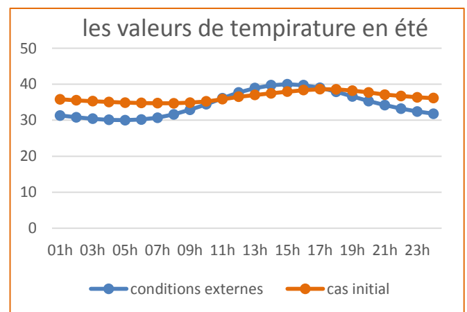
Figure 127: GRAPHE PRESENTE LES VALEURS DE LA TEMPERATURE EN ETE POUR LE CAS INITIALE
