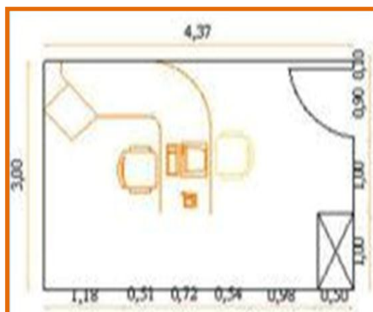
Figure 38: Dimensionnement Source : Neufert 8 ème Edition page 320 P
