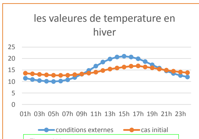
Figure 126: GRAPHE PRESENTE LES VALEURS DE LA TEMPERATURE EN HIVER POUR LE CAS
