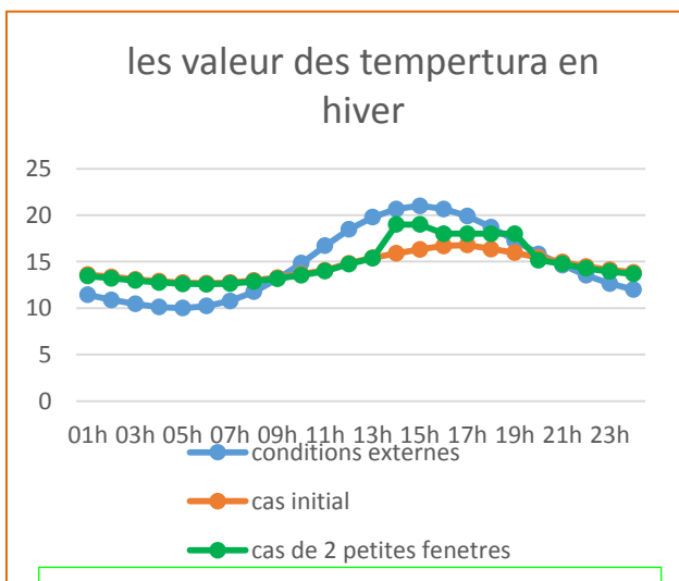
Figure 130: GRAPHE PRESENTE LES VALEURS DE LA TEMPERATURE EN HIVER POUR LE CAS AMELIORE N °2
