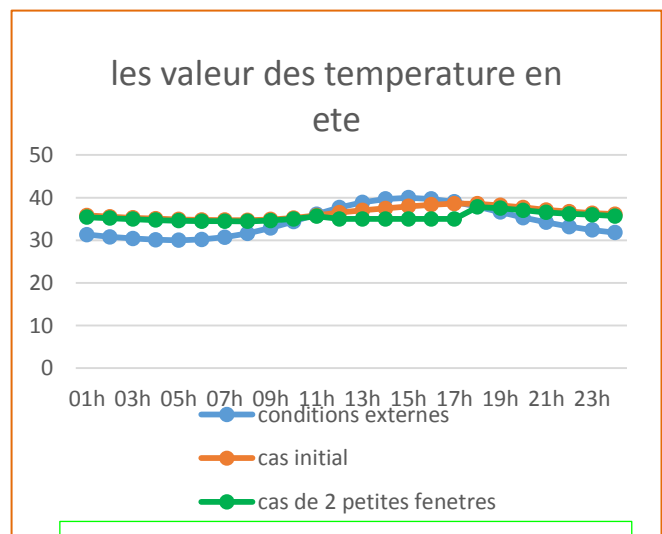
Figure 131: GRAPHE PRESENTE LES VALEURS DE LA TEMPERATURE EN ETE POUR LE CAS AMELIORE N °2
