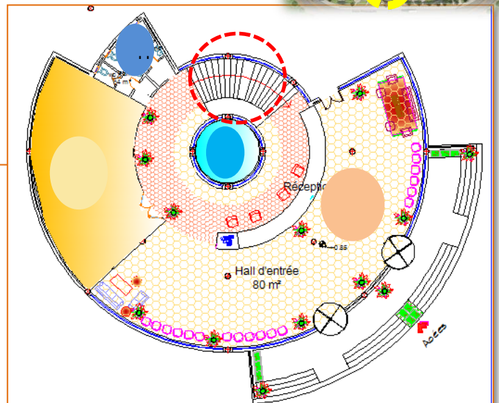
Plan RDC
