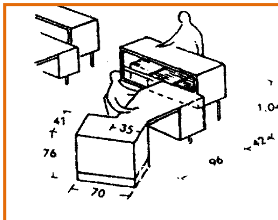
Figure 36: Dimensionnement Source : Neufert 8 ème Edition page 342
