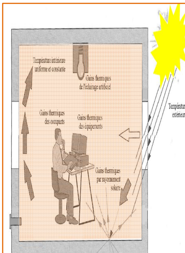
Figure 122 : GAIN THERMIQUE INTERNES D'UN ESPACE SOURCE :
