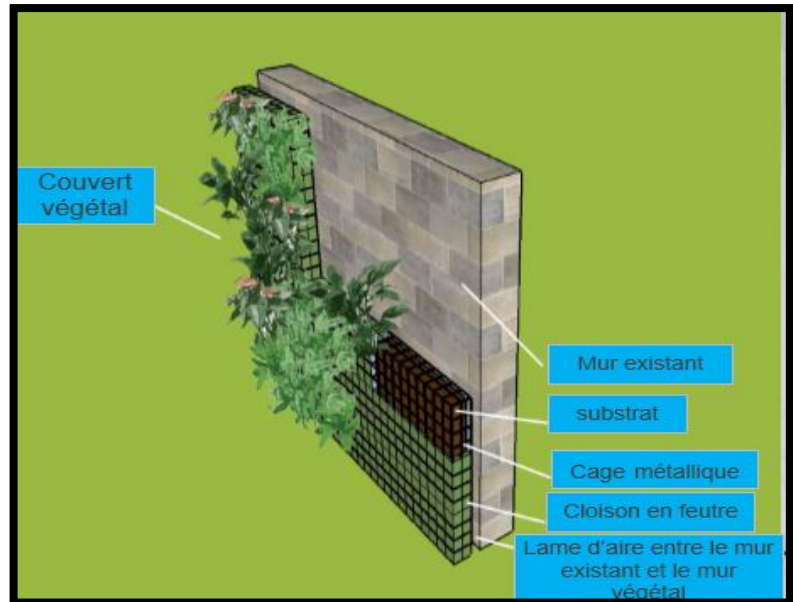
Figure 119 : les composantes de mur végétal
