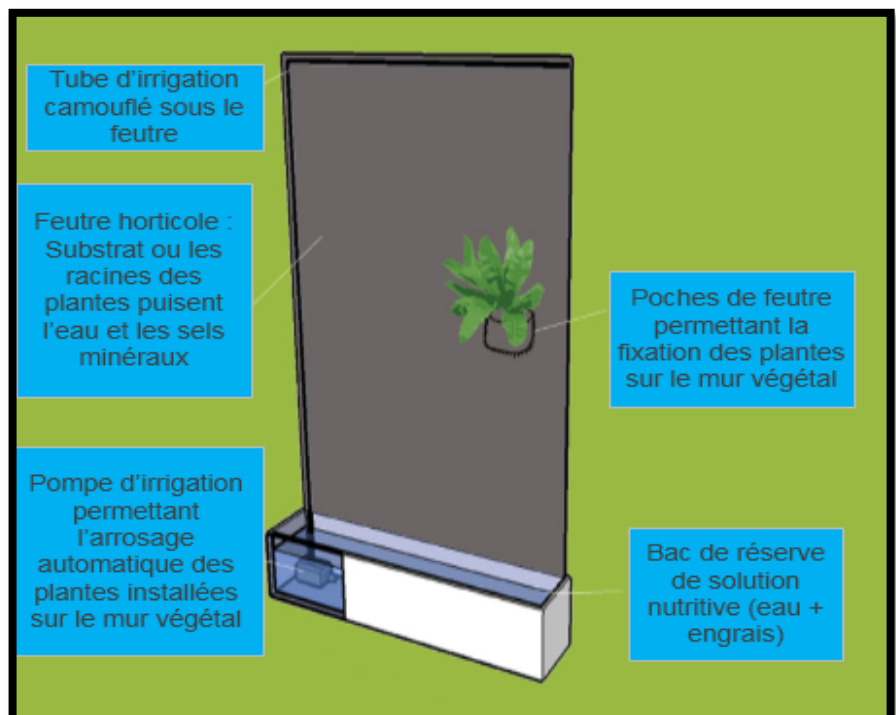
Figure 120 : détails de mur végétal
