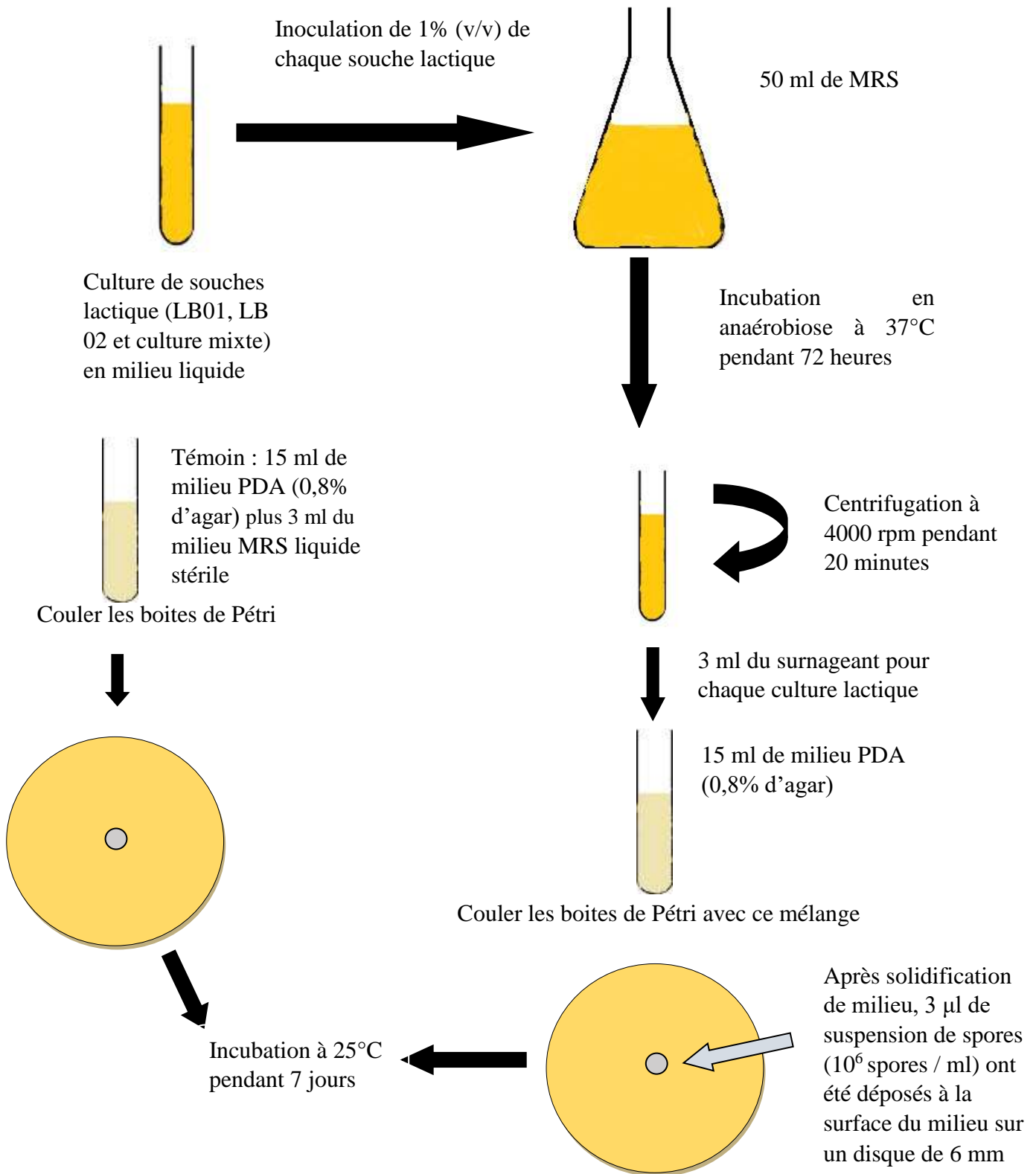
Figure 06 : Schéma représente les étapes de la mise en évidence de l'activité antifongique par la méthode de l'inhibition de croissance radiale (test qualitatif).
