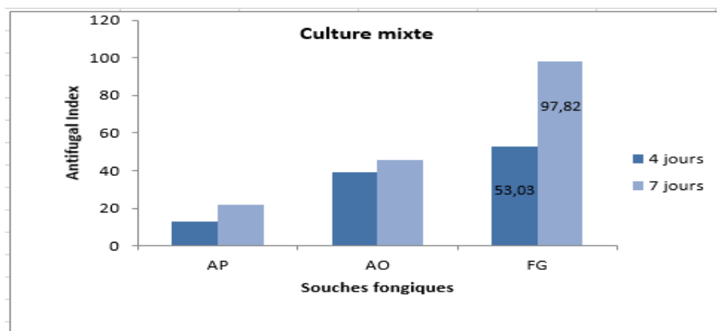
Figure 11 : Résultats de l'activité antifongique des souches Lactobacillus plantarum (LB01) et Lactobacillus acidophilus (LB02) en culture mixte sur la croissance radiale du mycélium des souches Fusarium graminearum (FG) ; Aspergillus ochraceus (AO) ; Aspergillus parasiticus (AP).
