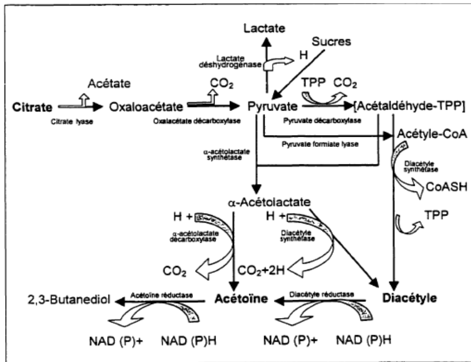
Figure 3 : Voie métabolique du citrate des lactocoques et leuconostocs citrate positif (Cit+) (Fox et al., 1990; Divies et al., 1991).
