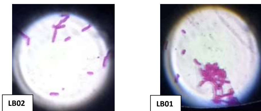
Figure 7 : Photos d'observation par microscope optique des cellules des bactéries lactiques après coloration de Gram (Objectif x100 à immersion) Lactobacillus plantarum (LB01) et Lactobacillus acidophilus (LB02)
