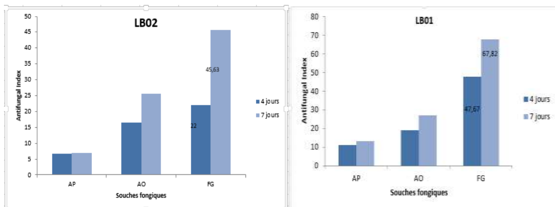
Figure 10 : Résultats de l'activité antifongique des souches Lactobacillus plantarum (LB01) et Lactobacillus acidophilus (LB02) sur la croissance radiale du mycélium des souches Fusarium graminearum (FG) ; Aspergillus ochraceus (AO) ; Aspergillus parasiticus (AP).
