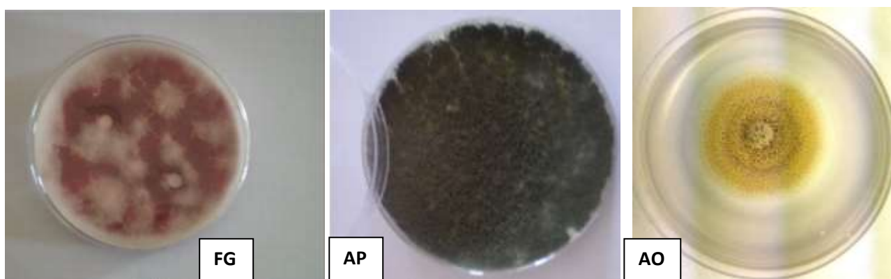
Figure 08: Photos d'observation macroscopique de l'aspect des cultures pures des souches fongiques sur milieu PDA. Gibberella zeae ( Fusarium graminearum ) (FG), Aspergillus ochraceus (AO) et Aspergillus parasiticus (AP)
