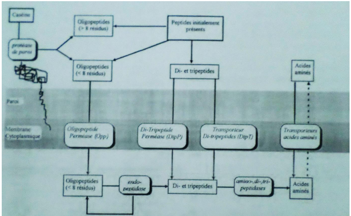
Figure02 : Utilisation des sources d'azote du lait par Lactococcus lactis (Juillard et al., 1996).
