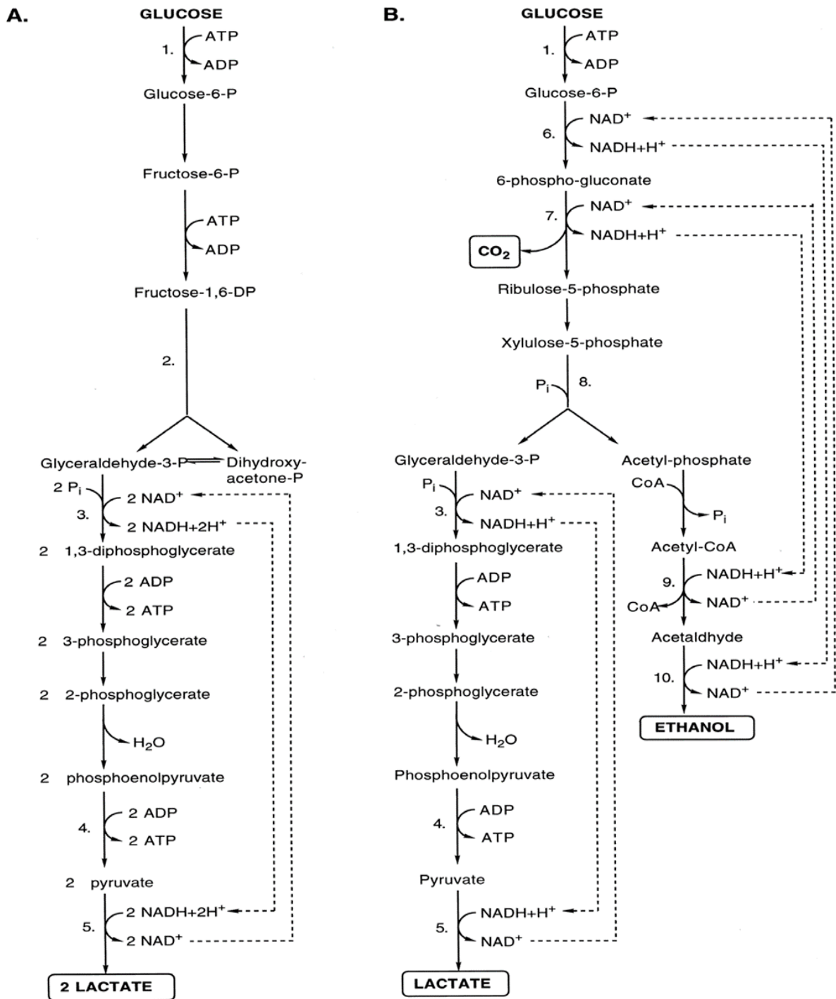
Figure 1 : Principales voies du métabolisme de glucose par les bactéries lactiques. (A) voie homofermentaire (B) voie hétérofermentaire (Thompson et Collins, 1989).
