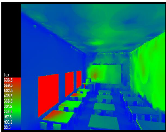
Figure 2.35: Niveau d'éclairément H. (Source : Auteurs)
