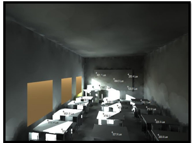
Figure 2.13 : Niveau d'éclairément H. (Source : Auteurs)
