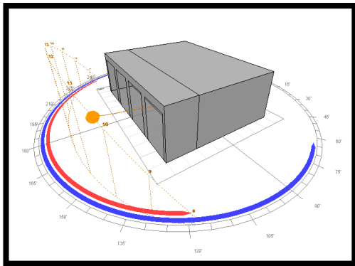
Figure 2.24 : L'ombre portée par le projet 21déc.
