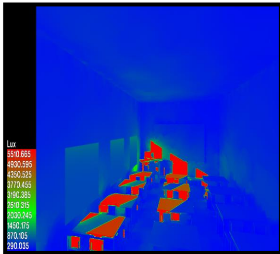
Figure 2.12 : Niveau d'éclairément H. (Source : Auteurs)
