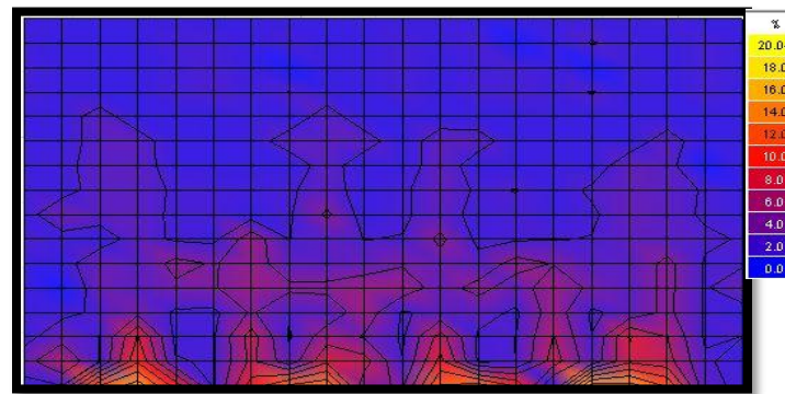
Figure 2.17 : facteur jour FLJ à 15 h 21 Décembre source : auteur
