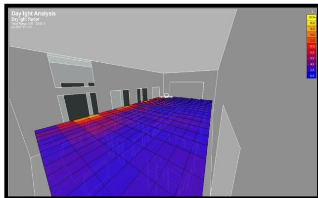
Figure 2.28: Niveau d'éclairément de jour FLJ
