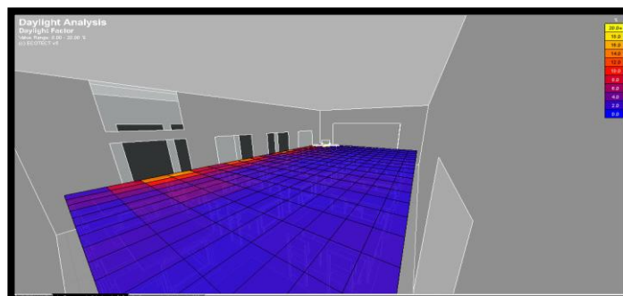
Figure 2.34 : Niveau d'éclairément de jour FLJ (Source : Auteurs)
