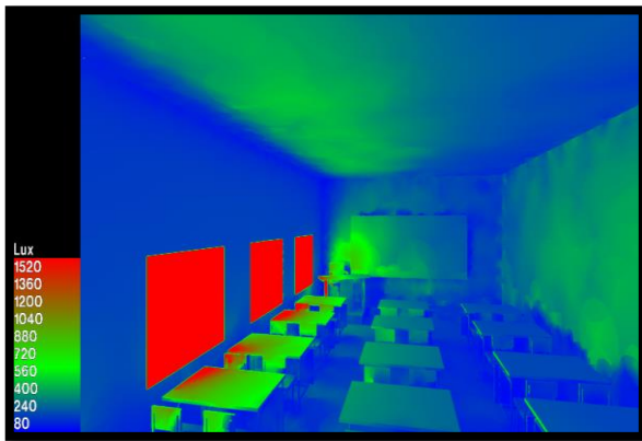
Figure 2.18 : Niveau d'éclairage H. et vertical (Source : Auteur)
