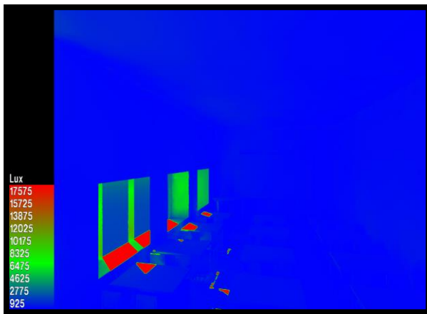
Figure 2.29: Niveau d'éclaircment H.
