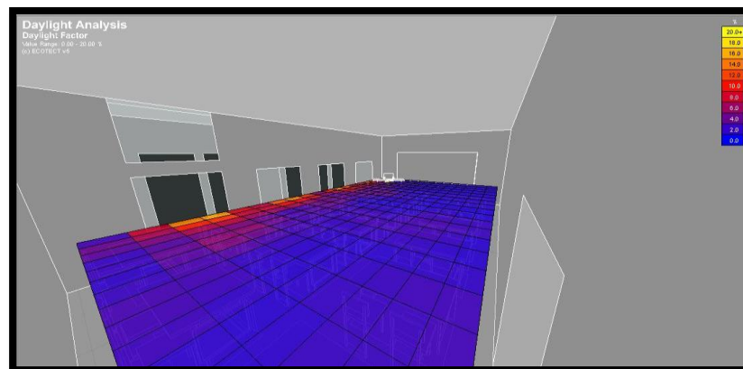
Figure 2.31 : Niveau d'éclaircment de jour FLJ
