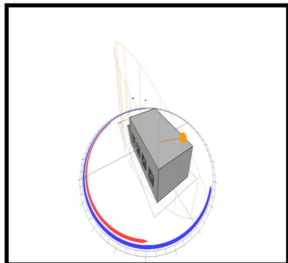
Figure 2.11 : L'ombre portée par le projet 21juin
