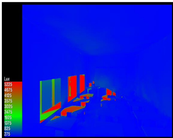
Figure 2.26: Niveau d'éclairément H.
