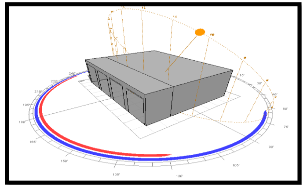
Figure 2.25 : L'ombre portée par le projet 21juin.
