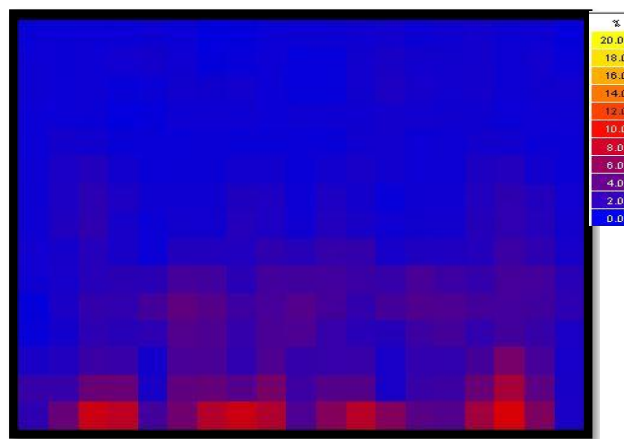
Figure 2.20: Niveau d'éclairage de jour FLJ (Source : Auteur)
