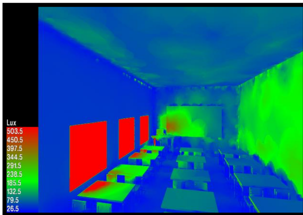
Figure 2.32: Niveau d'éclairément H. (Source : Auteurs)
