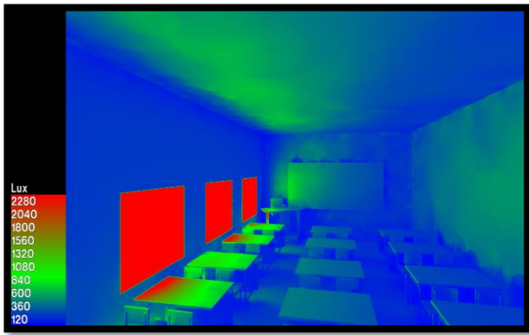
Figure 2.21 : Niveau d'éclairément H. (Source : Auteurs)
