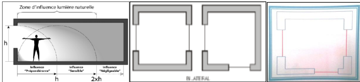
Figure V 7: Les types d'éclairage latéral.
