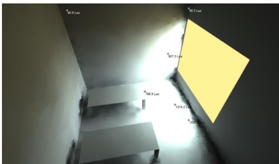
Figure V 25: Vue Intérieure à 12 h Source : Auteurs
