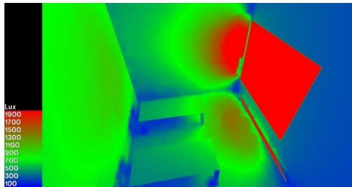
Figure V 23: Niveau D'éclairage en false colore Source : Auteurs
