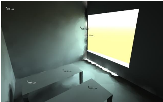
Figure V 18: Vue Intérieure à 12 h Source : Auteurs
