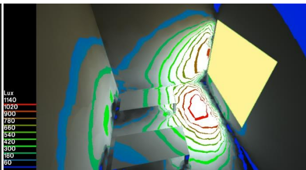
Figure V 24: Niveau D'éclairément en Contour Ligne Source : Auteurs
