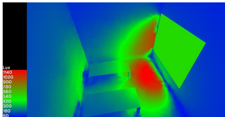
Figure V 26: Niveau D'éclairément en false colore Source : Auteurs
