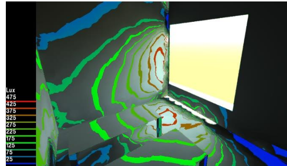
Figure V 19: Niveau D'éclairéement en Contour Ligne Source : Auteur
