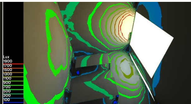
Figure V 22: Niveau D'éclairage en Contour Ligne Source : Auteur
