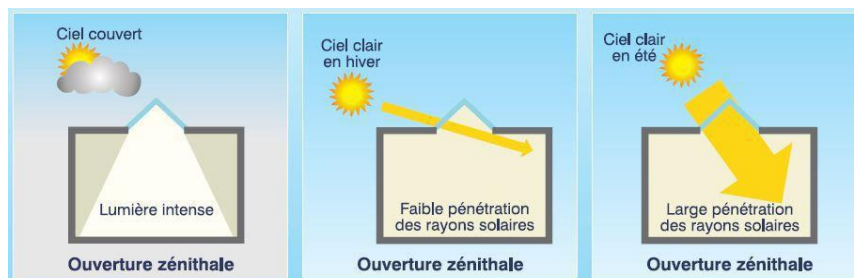
Figure V 8 : Dispositifs les types es des ouvertures zénithale ; Source : (Liébard, A. et De Herde, A., 2005)
