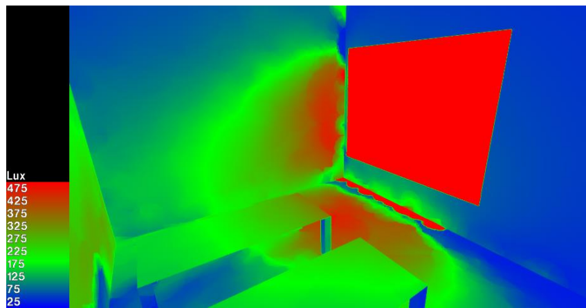
Figure V 20: Niveau D'éclairéement en false colore Source : Auteurs
