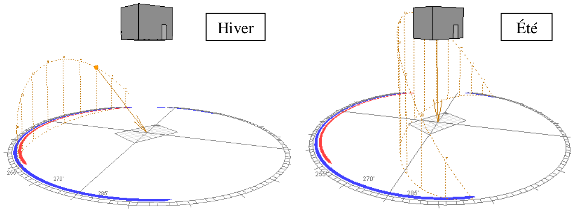
Figure 1e diagramme solaire Cas d'été et cas hiver Source : Auteurs
