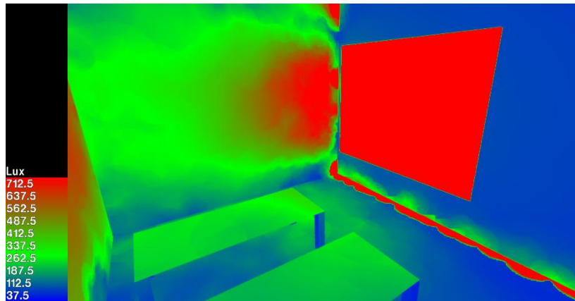
Figure V 17:Niveau D'éclairage en false colore Source : Auteurs
