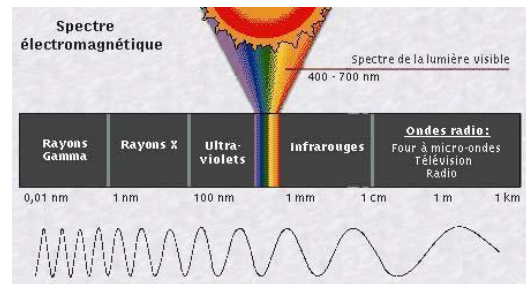
Figure V 5 : Spectre électromagnétique. [champo- tpe.e-monsite.com].
