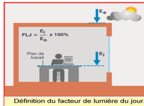
Figure V 2: Définition de facteur de lumière de jour. [Source : http://www.vizea.fr ]
