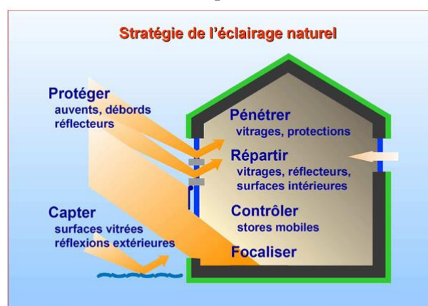
Figure V 9 : Stratégie de la lumière naturelle. [Source : l'architecture t et climat].
