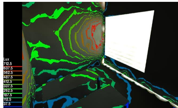
Figure V 15: Niveau D'éclairage en Contour Ligne Source : Auteurs
