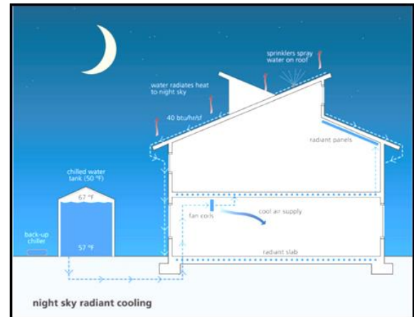
Fig.II-48 Refroidissement radiant [Source : http://deg.stanford.edu/about/building ]
