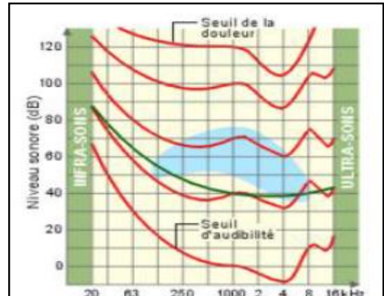
Fig. VI-37 la courbe d'évaluation du bruit Source: énergie plus.com
