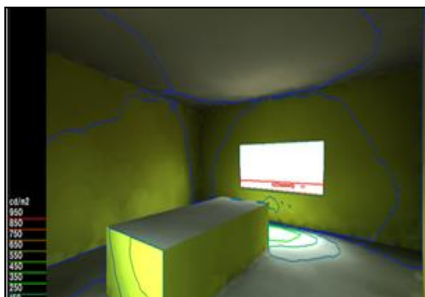
Fig. VI-12. courbe iso à ciel couvert [Source : l'auteur / radiance]
