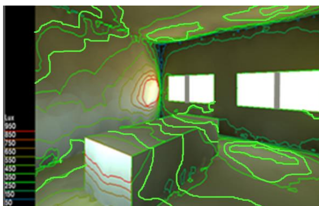
Fig.VI-25 Courbe iso à ciel clair [source : l'auteur / radiance]
