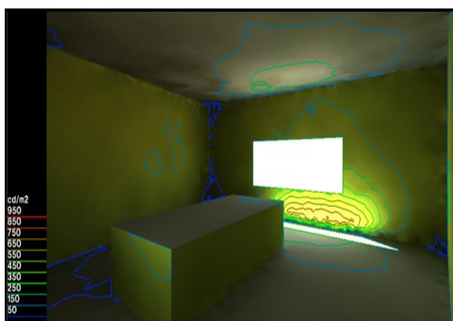
Fig.VI-20.Courbe iso à ciel clair [Source : l'auteur / radiance]
