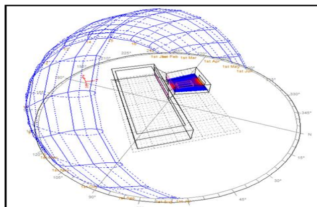
Fig. VI.14. Niveau d'éclairage à l'intérieur [Source : auteur / ecotect]
