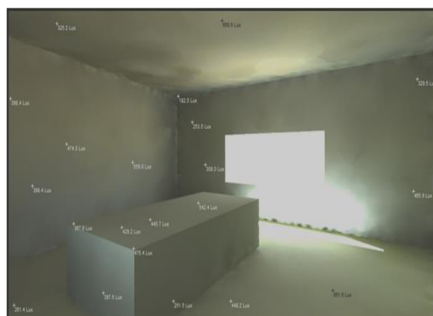
Fig.VI-21.Mesure de niveau d'éclairage à des points différents à ciel clair [Source : Auteur/ radiance]
