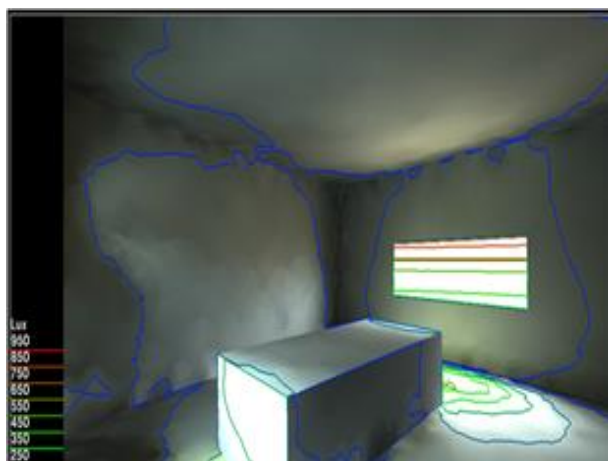
Fig.VI-15. Contour de FLJ [Source : auteur / écotect]
