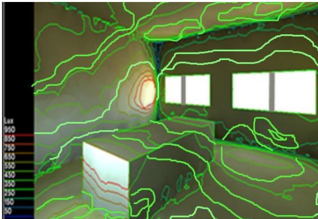
Fig.VI-27. courbe iso à ciel clair Source : l'auteur / radiance
