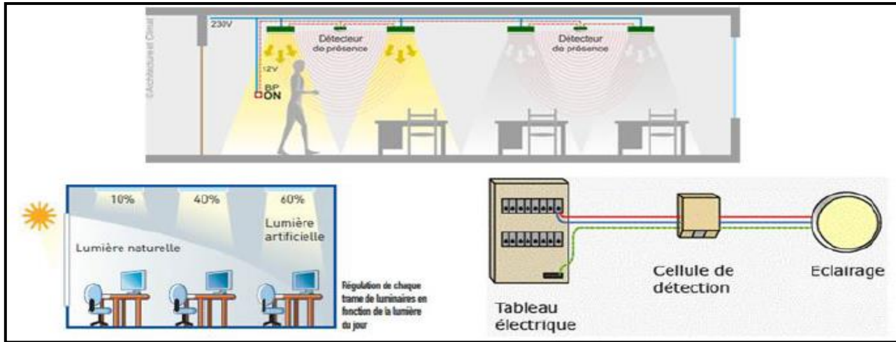
Fig. VI-43. schéma de fonction de détecteur de présence dans l'éclairage
