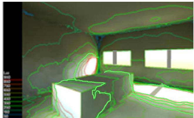
Fig.23. Niveau d'éclairage à l'intérieur [Source : auteur / ecotect]
