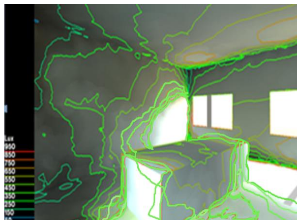
Fig.24. Niveau d'éclairement à l'intérieur Source : auteur / écotect
