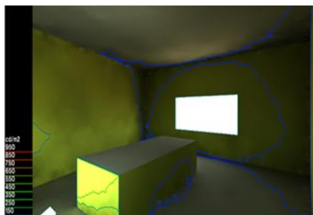
Fig.VI-17 Courbe iso à ciel clair [Source : l'auteur / radiance]
