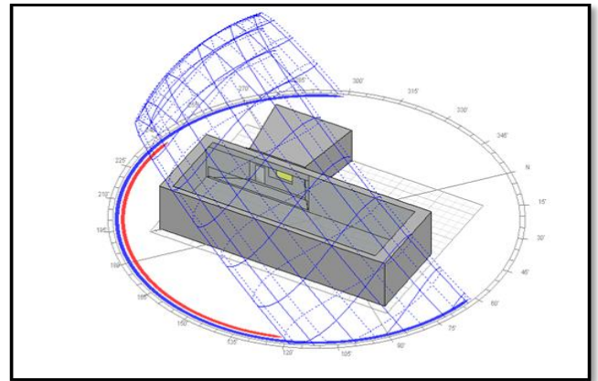
Fig.VII-09. Espace étudié [Source : auteurs / ecotect]
