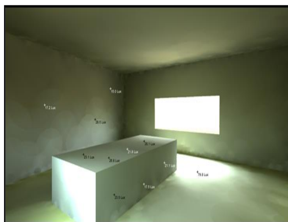
Fig. VI-13. Mesure de niveau d'éclairage à des points différents à ciel couvert [Source : Auteur/ radiance]
