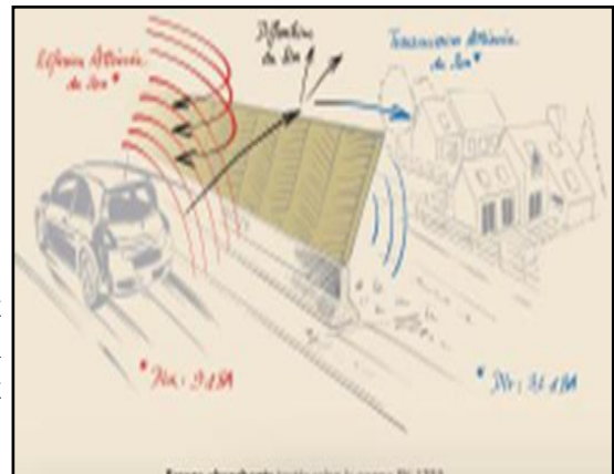
Fig. VI-38 écran acoustique absorbant [Source: www.tertu.com]
