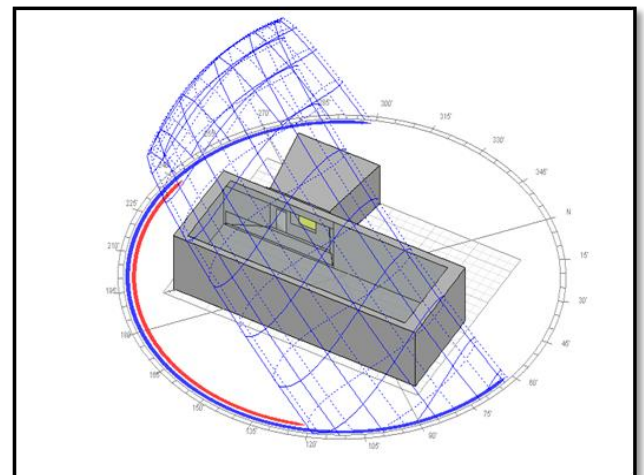
Fig.VI-22. L'espace de simulation cas d'amélioration [Source : auteurs / ecotect]
