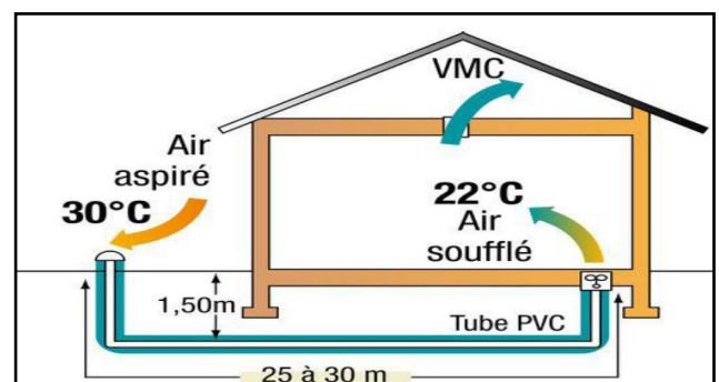
FigI.16 Puits canadien [Source : novation écologique, Transformer sa maison au naturel : isoler, restaurer]
