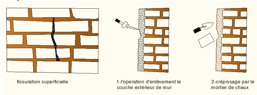
Figure171 III : traitement de fissuration élaborer par les étudiantes
