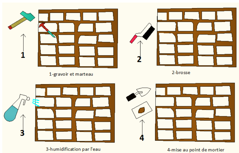
Figure 170 III: traitement L érosion de la pierre élaborer par les étudiantes
