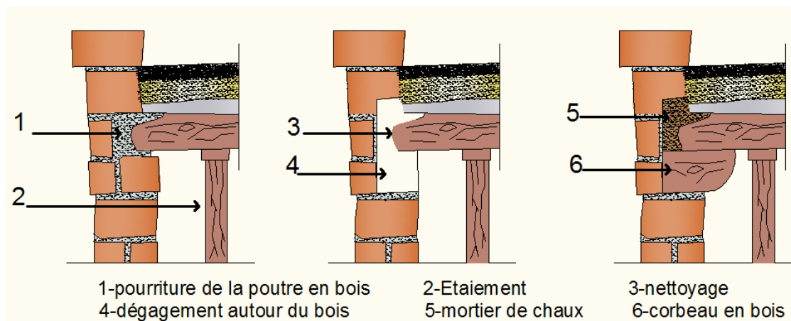
Figure 166 III : Les étapes de restauration des plancher élaborer par les étudiantes
