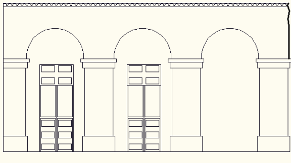
Figure 164 III: les arcades délabrées avant la reconstruction élaborer par les étudiantes
