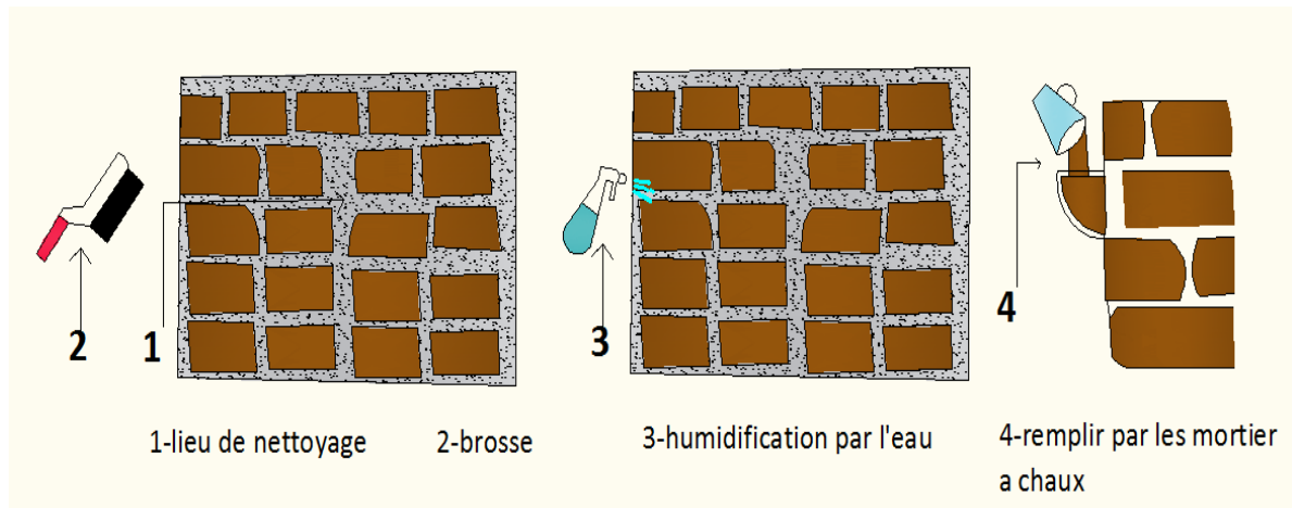
Figure169 III: traitement de dégradation des mortiers élaborer par les étudiantes
