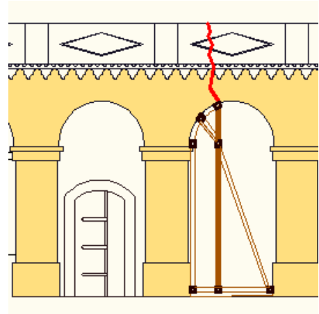
Figure 146 III : l'étaiement proposé élaborer par les étudiantes
