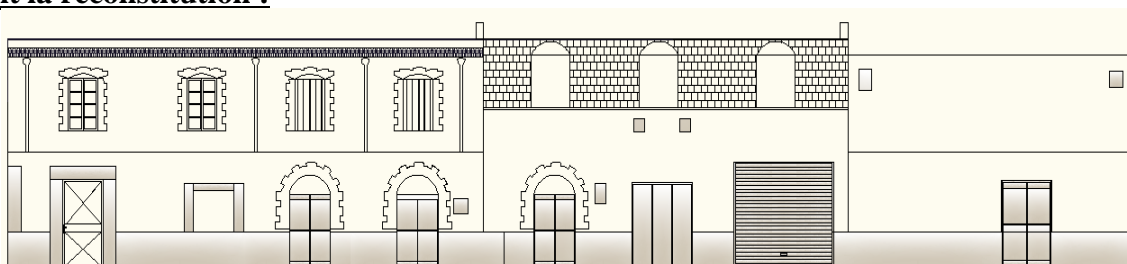
Figure 174 III : la façade nord de la place de l'étoile élaborer par les étudiantes
