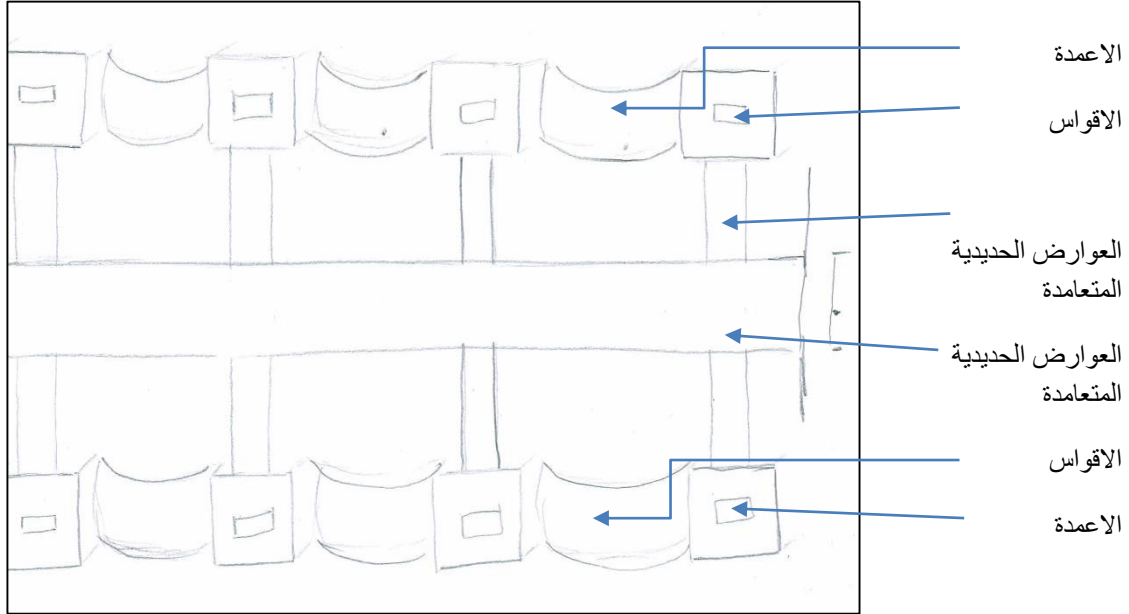
الوثيقة -33- رسم توضيحي لتدعيم السقف (انجاز الطالب)
