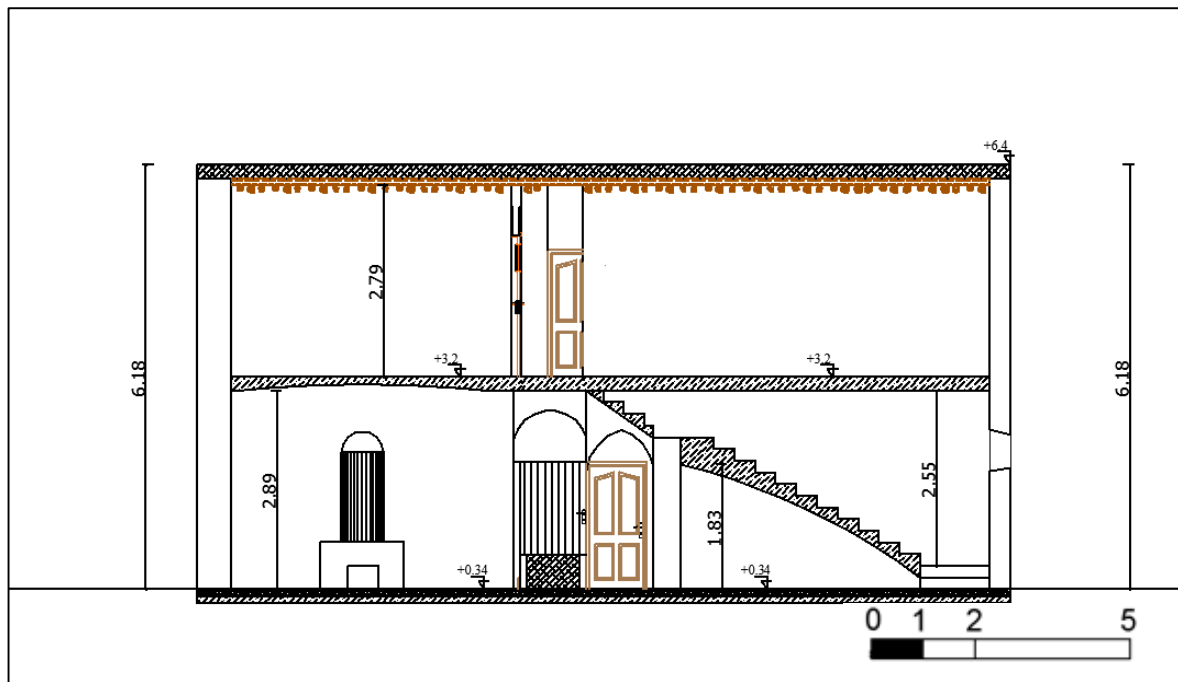
الوثيقة -25- مقطع مسجد التاوتي (انجاز الطالب)
