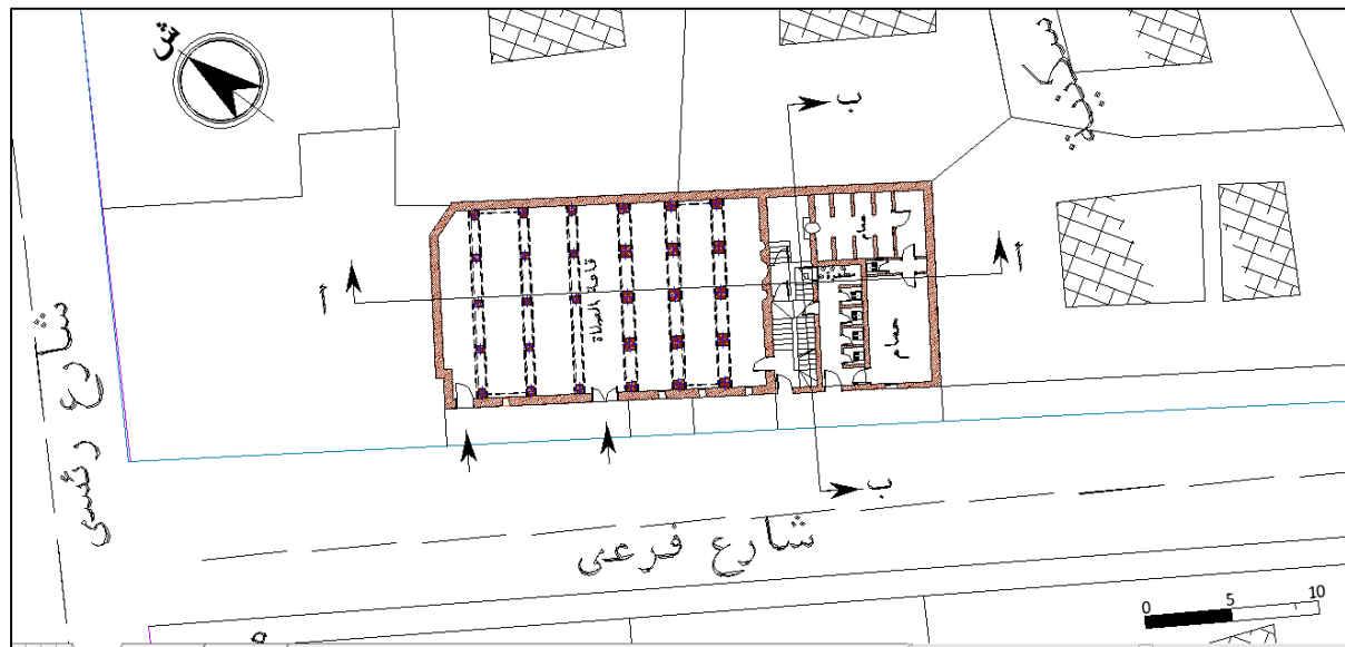
الوثيقة-26- مخطط الطابق الأرضي للمسجد بعد التحول (انجاز الطالب)
