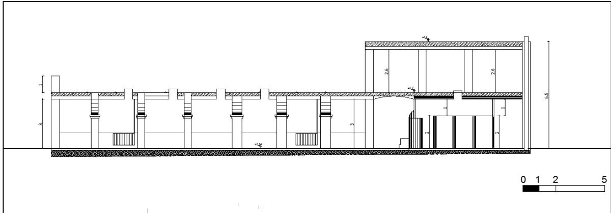
الوثيقة -29- مقطع أ-أ للمسجد بعد التحول (انجاز الطالب)
