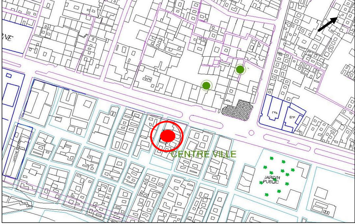
وثيقة 16- مخطط موقع مسجد التاوتي (توظيف الطالب)
