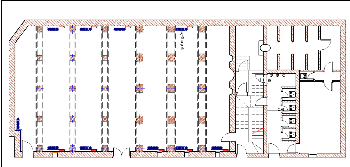
الوثيقة -30- مخطط التدفئة مسجد التاوتي (انجاز الطالب)
