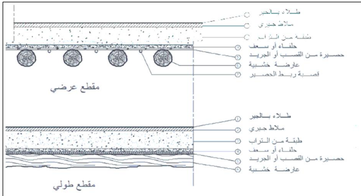
الوثيقة -34- مقطع عرضي وطولي لتركيب سقف تقليدي (التخي بلقاسم)
