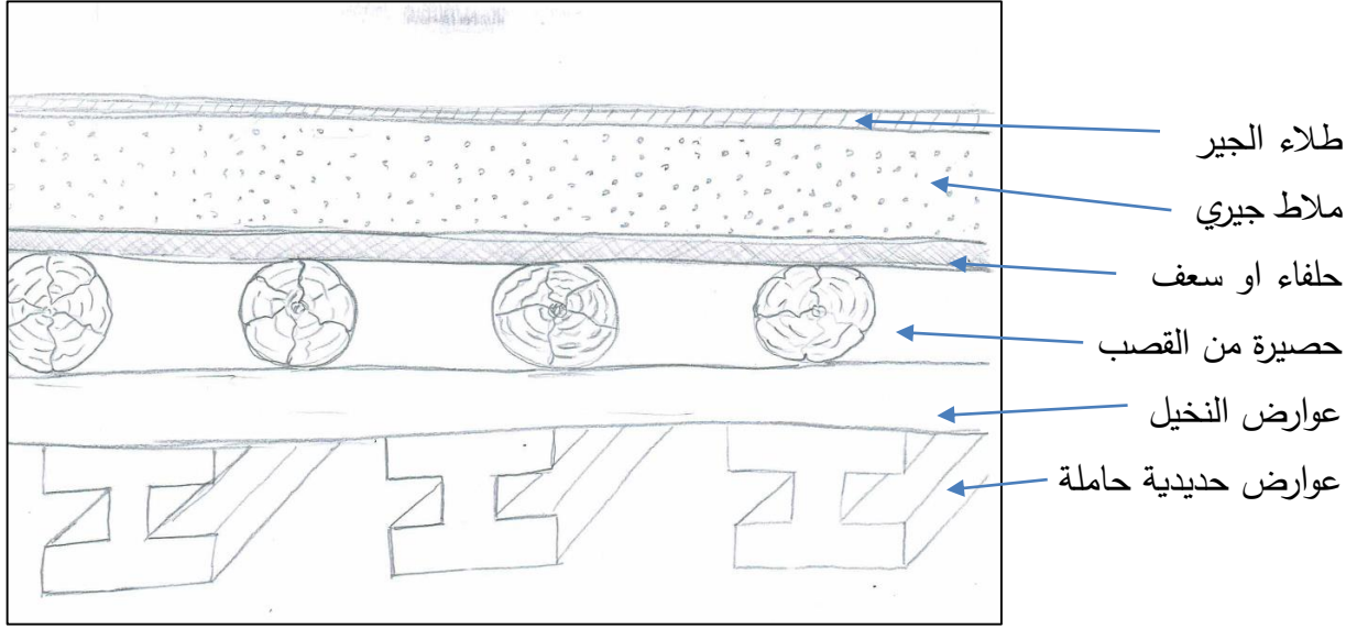
الوثيقة -32- رسم توضيحي لتدعيم السقف (انجاز الطالب)
