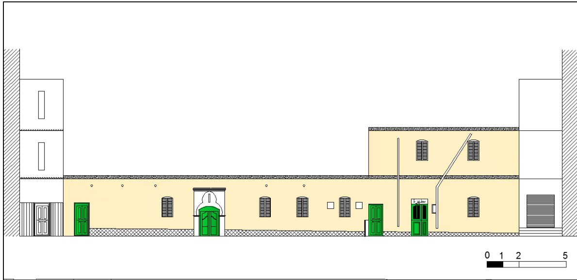
الوثيقة -28- مخطط واجهة المسجد بعد التحول (انجاز الطالب)
