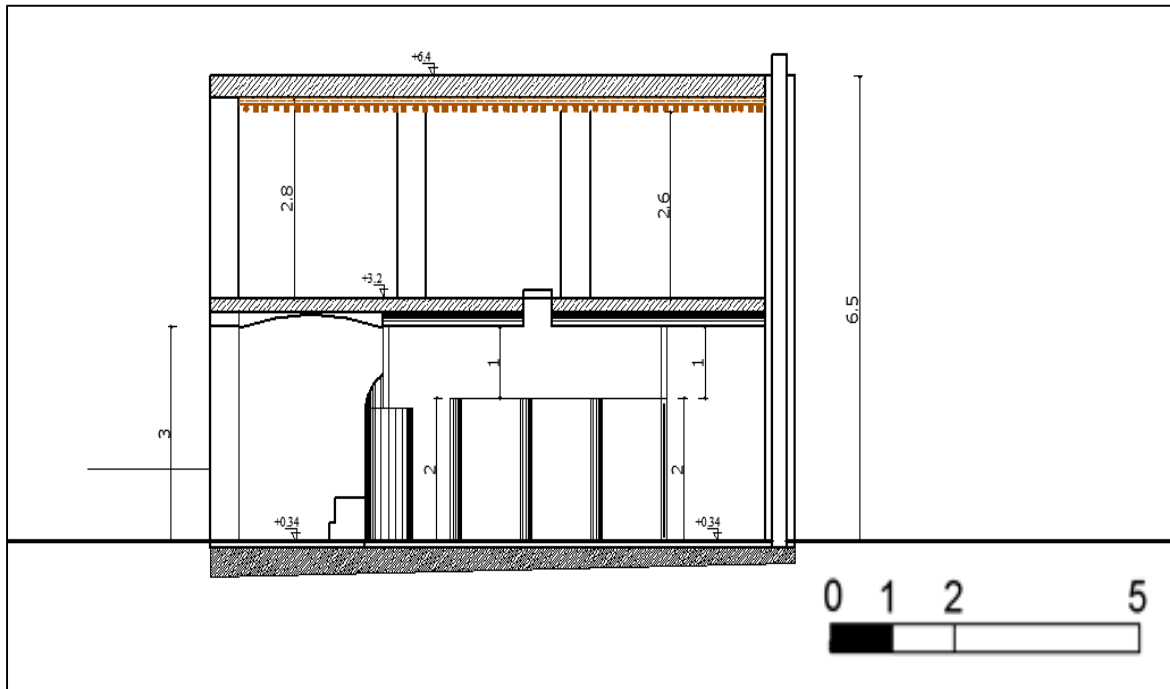
الوثيقة -24- مقطع حمام مسجد التاوتي (انجاز الطالب)
