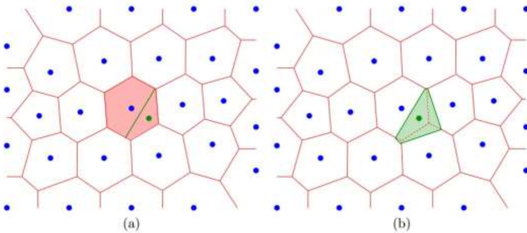
Figure 10 Constriction incrémentale de diagramme voronoi
