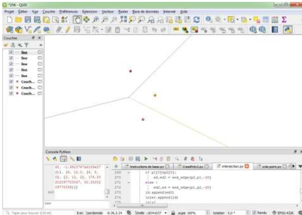
Figure 15. diagramme de voronoi pour 3 points
