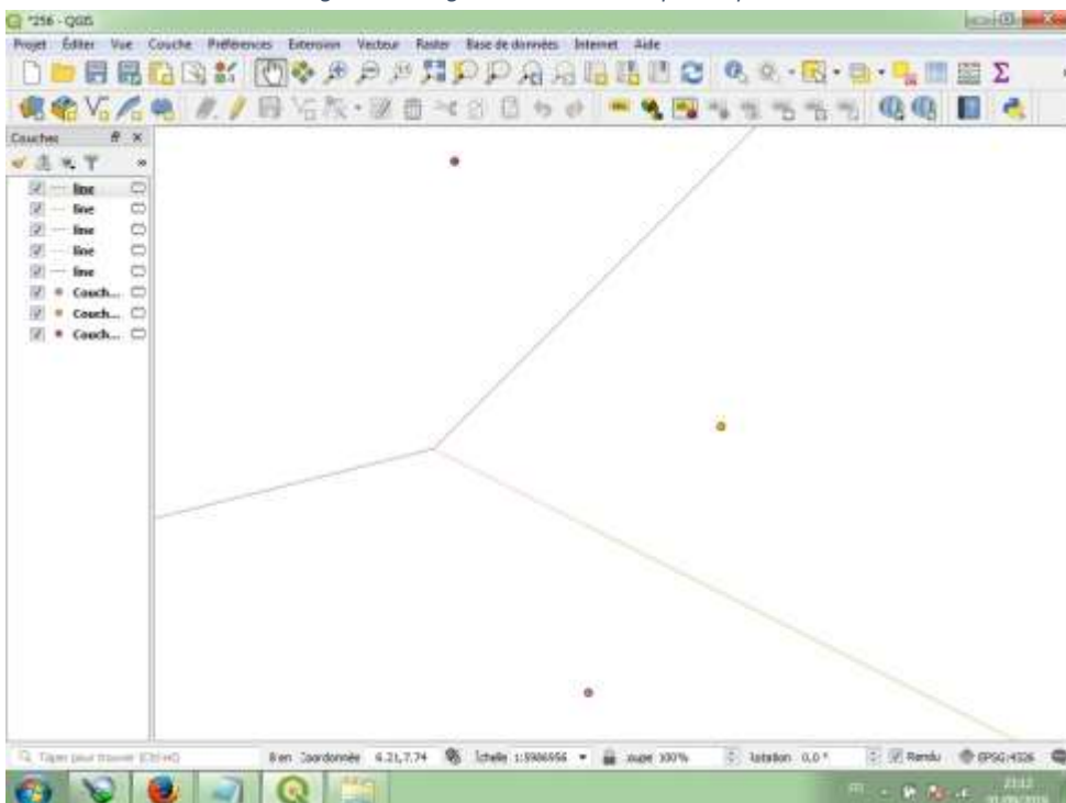
Figure 16. diagramme de voronoi pour 3 points différents
