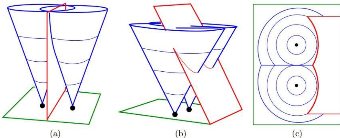
Figure 12 – Algorithme de Fortune. (a) L'intersection de deux cônes se projette sur la médiatrice [12]
