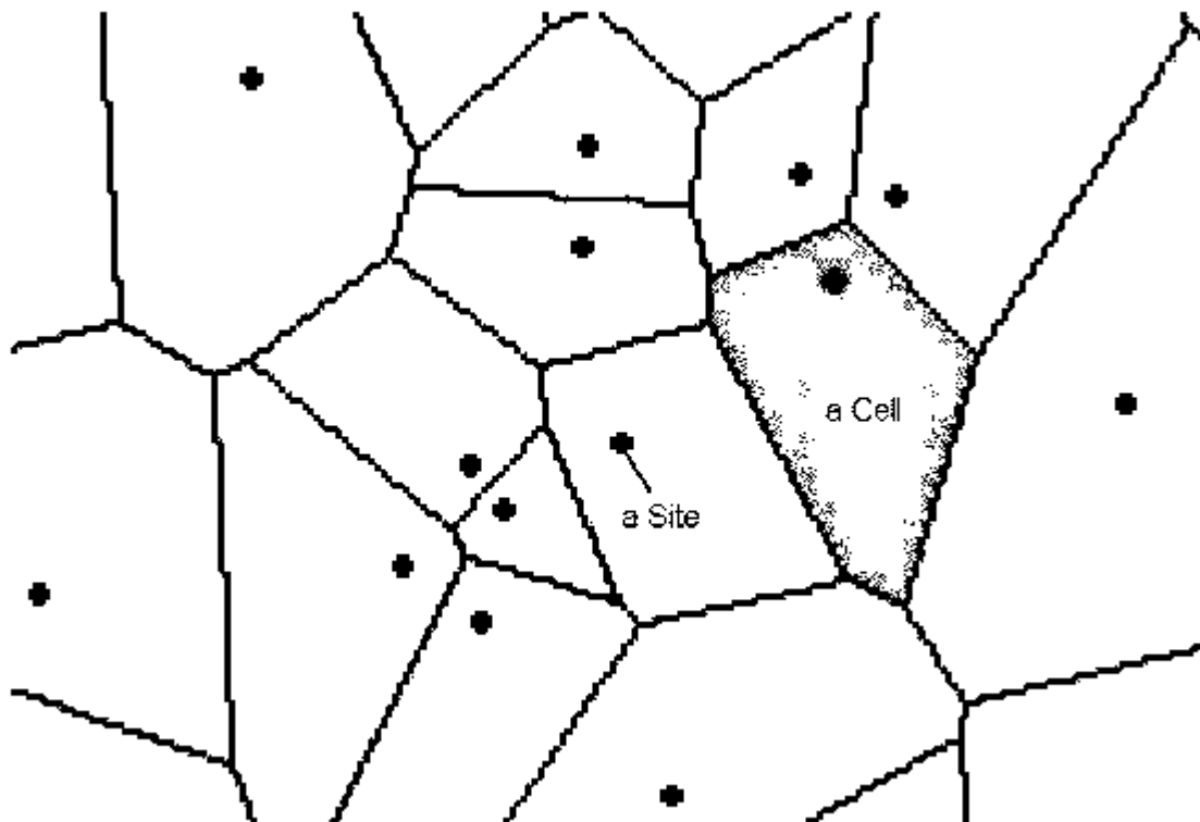
Figure 8. Diagramme de Voronoi
