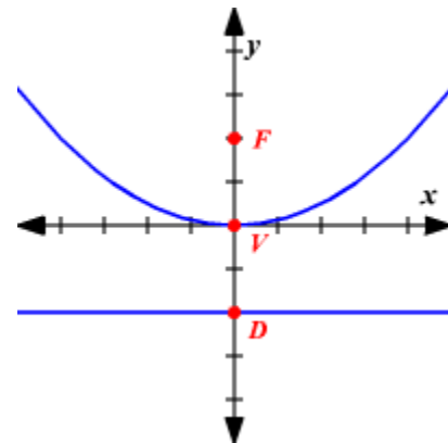
Figure 14. Relation entre le foyer, le sommet et la directrice
