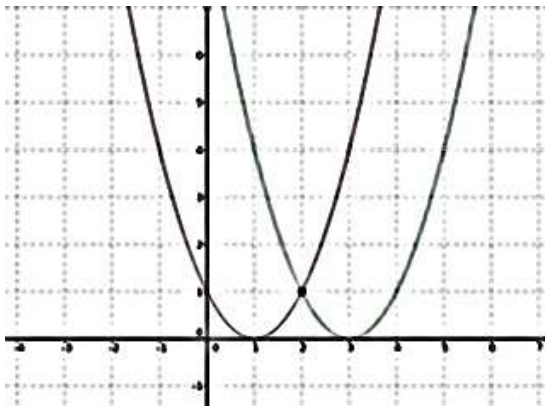
Figure 13. Deux paraboles
