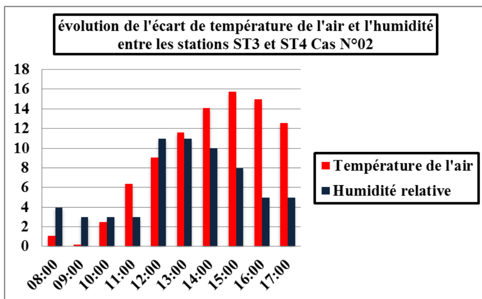
Figure IV. 19 : évolution de l'écart de température de l'air et l'humidité entre les stations ST3 et ST4 cas N°02. Source : auteur.
