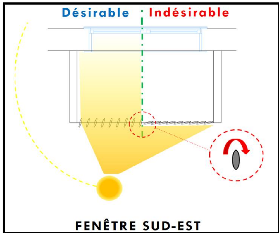
Figure V. 42 : Schéma pour les stores utilisés. Source : auteur.
