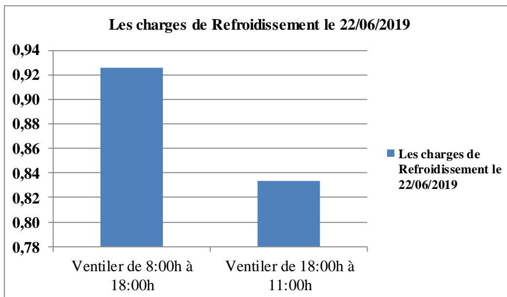
Figure IV. 46 : Les Charges de refroidissements. Source : auteur.
