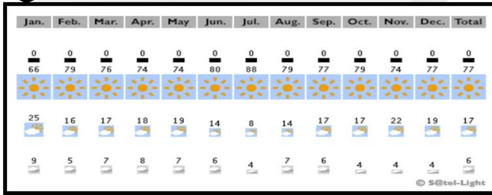
Figure III. 6 : Fréquence des ciels ensoleillés, intermédiaires et nuageux. Source : www.satel-light.com.
