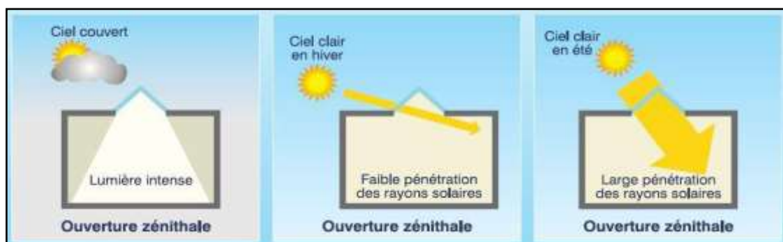
Fig IV.17 : Dispositifs les types des ouvertures zénithale ;Source (Liébard, A. et De Herde, A., 2005)
