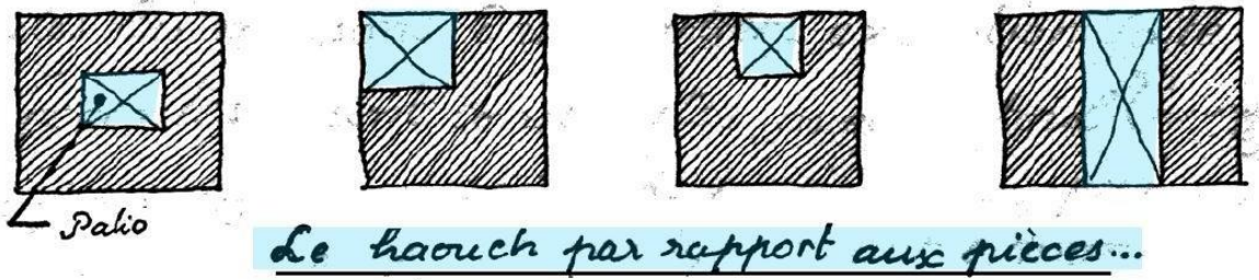
FIG25. ORGANISATION DES DIFFERENTES PIECES AUTOUR DU PATIO « HAOUCH »
