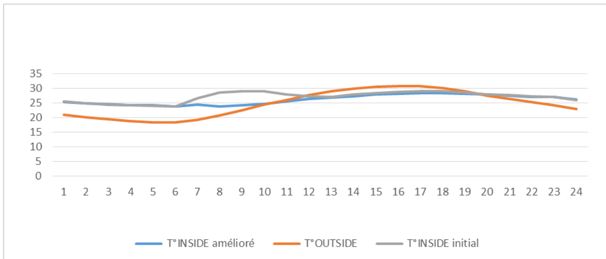
Figure 166: Graphe qui représente la déférence de cas initial et cas amélioré en été. Source : auteur.
