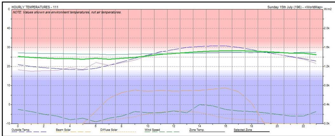
Figure 164: graphe qui représente la température du cas amélioré en été source : le logiciel écôtent adaptée
