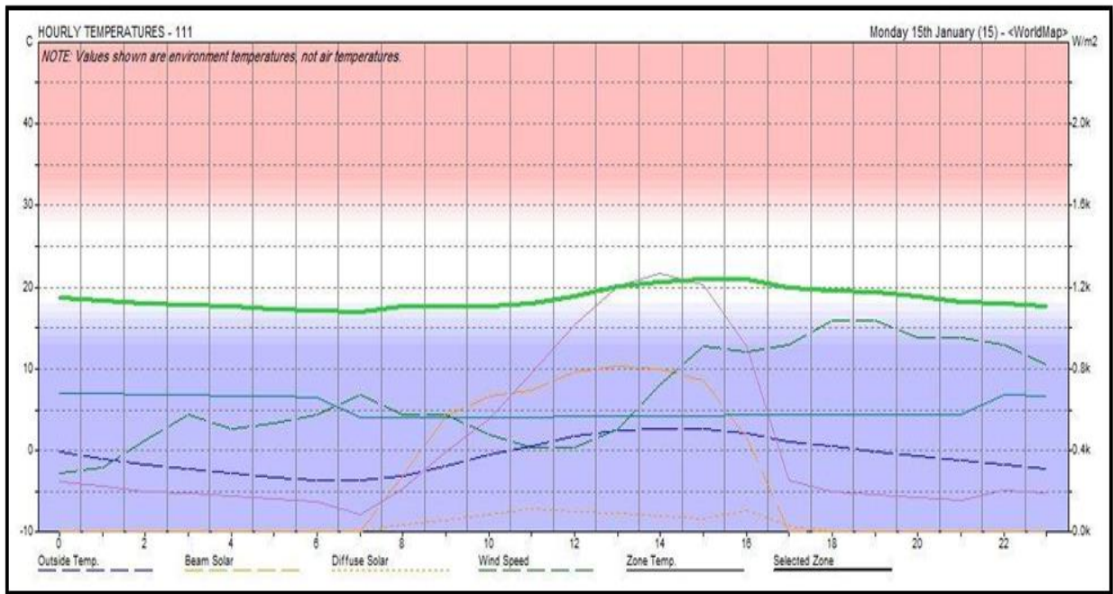
Figure 162: graphe qui représente la température du cas amélioré en hiver .Source : le logiciel écôtent adaptée auteur.
