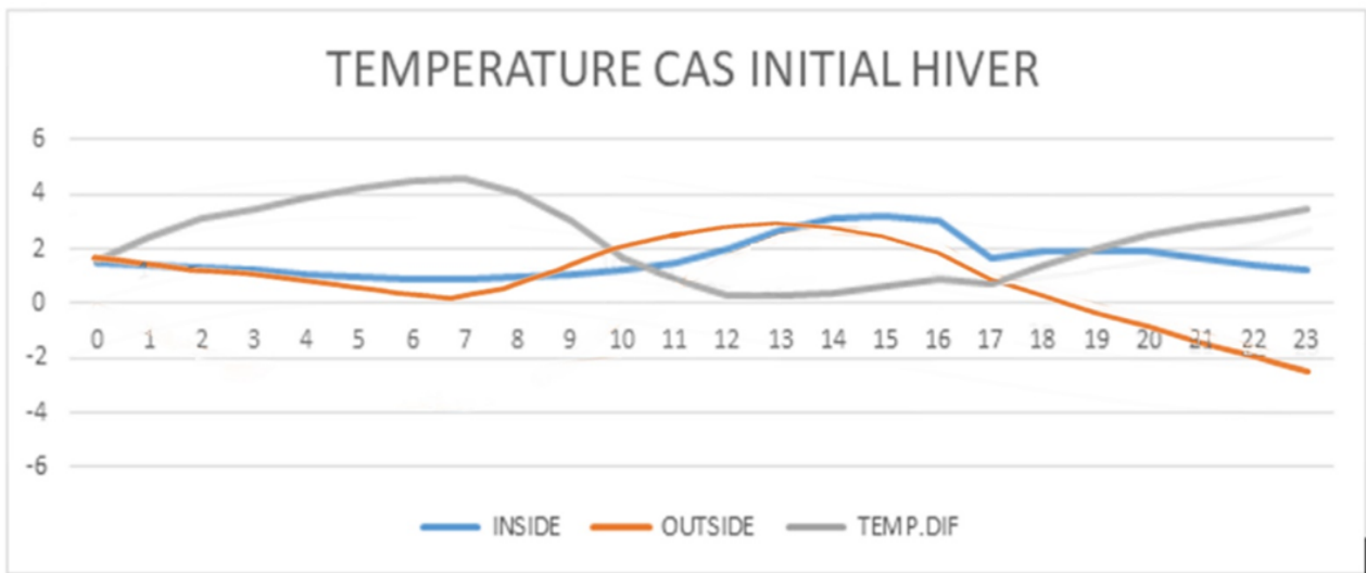
Figure 158; graphe qui représente les températures du cas initial en hiver .Source : auteur.
