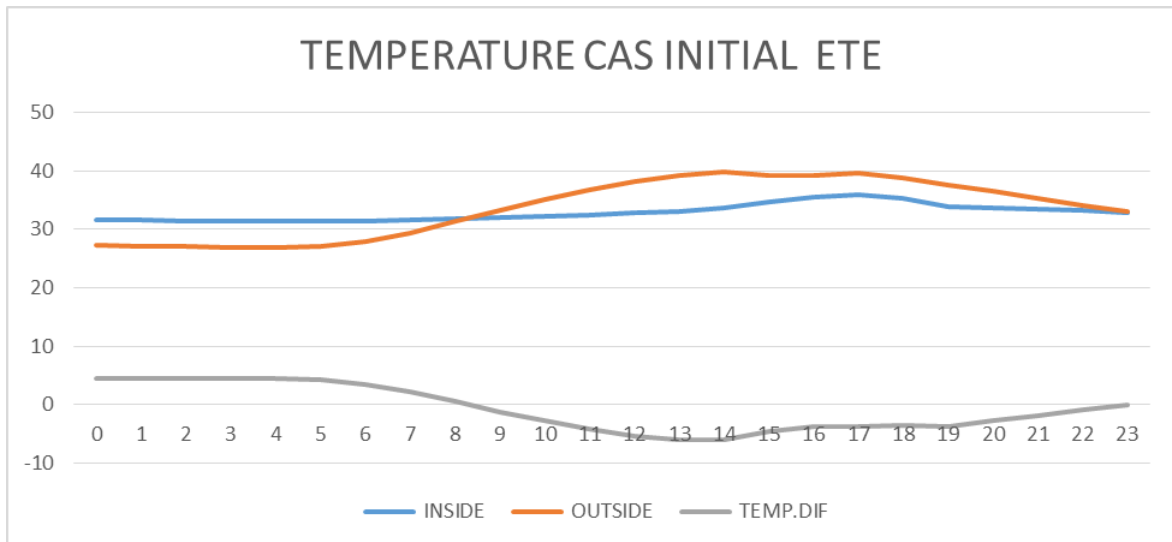
Figure 160: graphe qui représente les températures du cas initial en hiver .Source : auteur.
