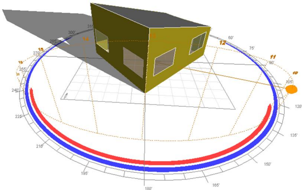
Figure 153: vue 3d de cas initial en hiver. Source : auteur.
