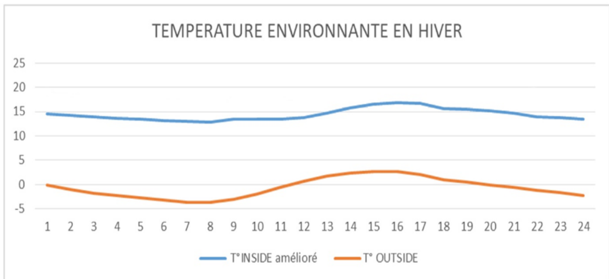
Figure 163: graphe qui représente la température du cas amélioré en hiver. Source : auteur
