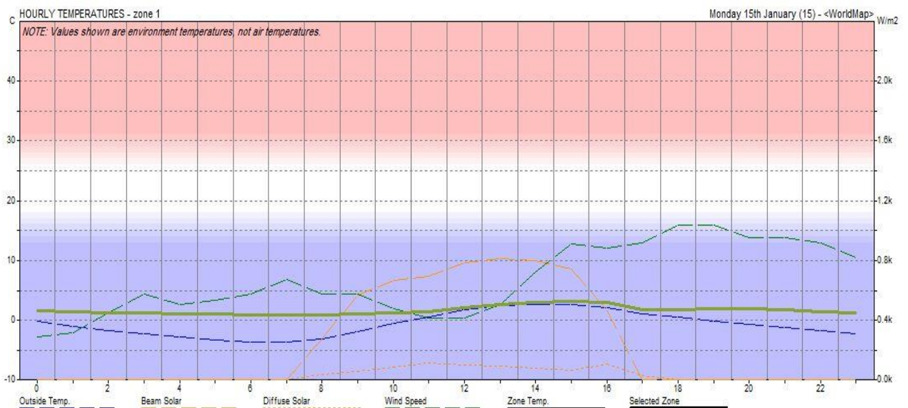
Figure 157:graphe qui représente la température du cas initial en hiver. Source : le logiciel ECOTEC adaptée auteur.
