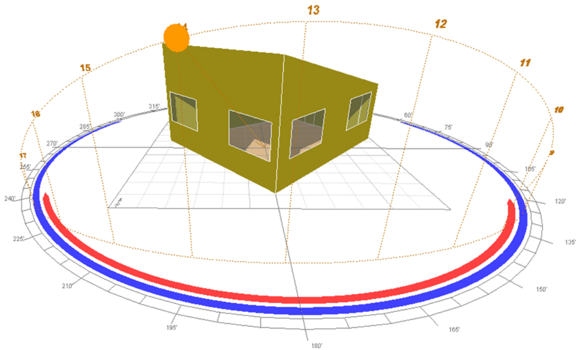
Figure 154 : vue 3d de cas initial en hiver. Source : auteur.
