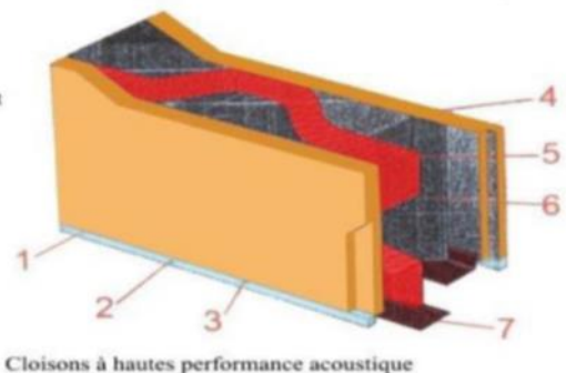
Cloisons à hautes performance acoustique Figure 133:Mur avec isolation acoustique. Source : www.cloisonsabesoinsperformanceacoustique.com .
