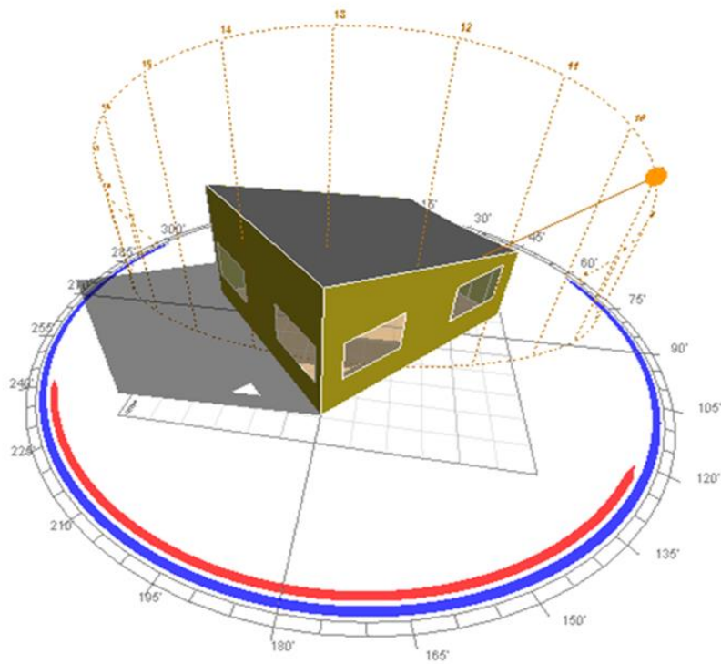
Figure 155:vue 3d de cas initial en été. Source : auteur.
