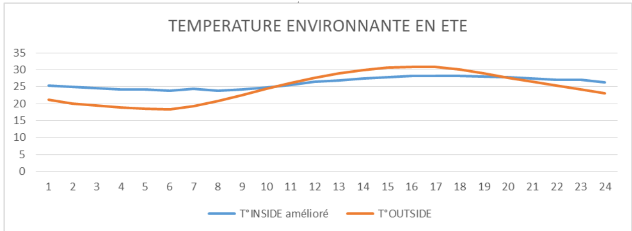
Figure 165: graphe qui représente la température du cas amélioré en été .Source : auteur
