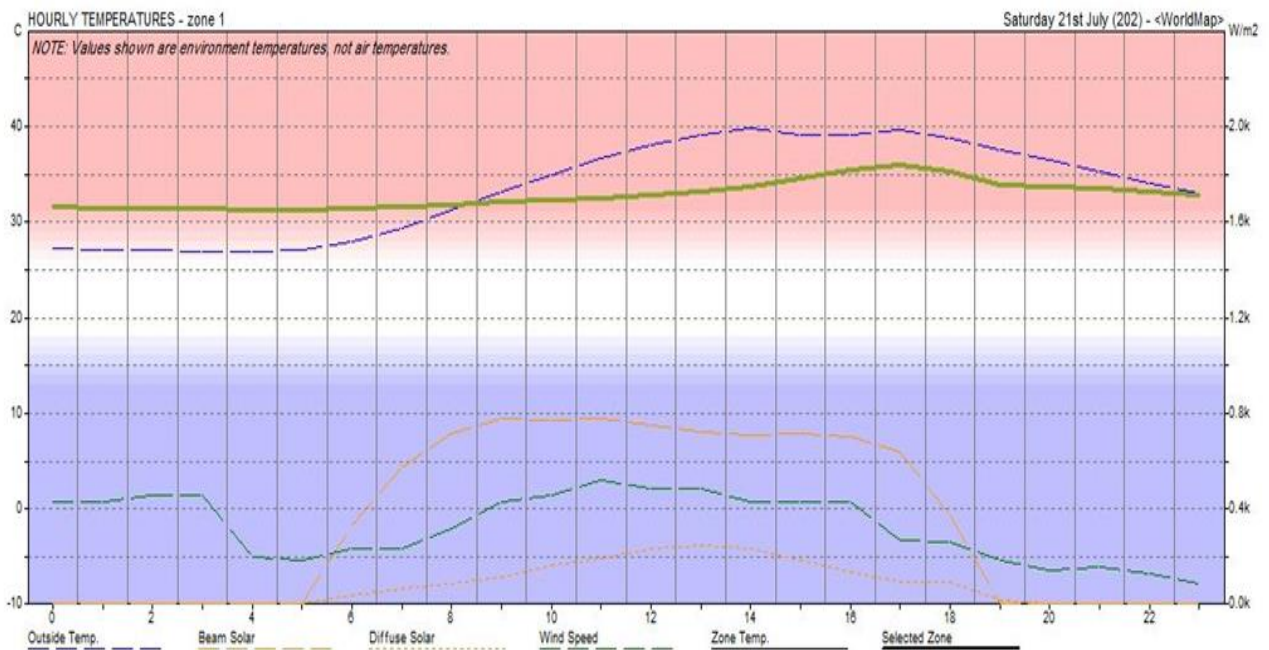
Figure 159: graphe qui représente la température du cas initial en été. Source : le logiciel ECOTEC adaptée auteur.
