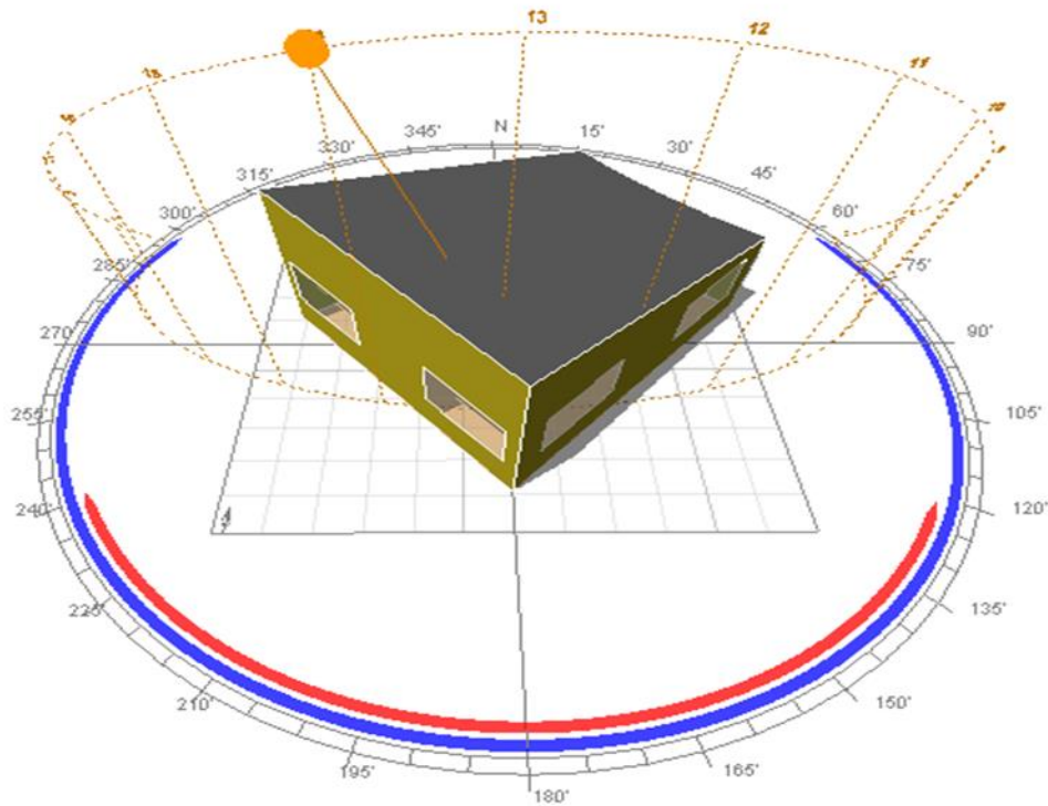
Figure 156:vue 3d de cas initial en été. Source : auteur.
