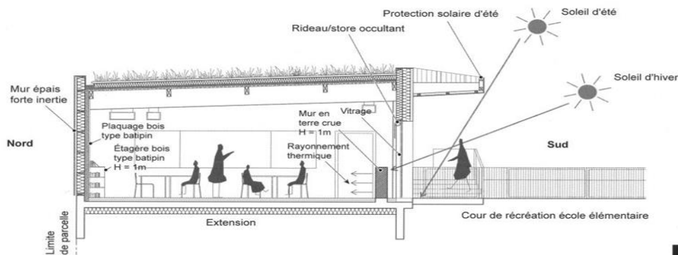
Figure 49 : prise en compte des apports solaires et mise en place de protections solaire /source : De la « maison d'école » au groupe scolaire B.B.C. Evolution de l'institution et de ses locaux les bâtiments scolaire contexte et enjeux locaux "6 octobre.
