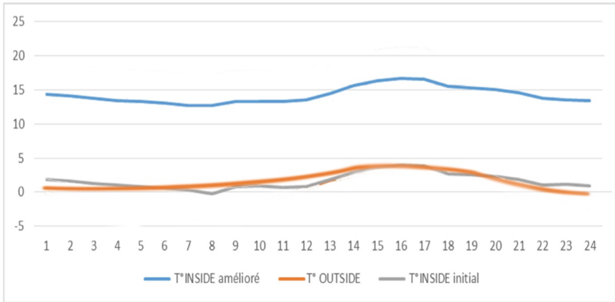
Figure 167: Graphe qui représente la déférence de cas initial et cas amélioré en hiver Source : auteur.
