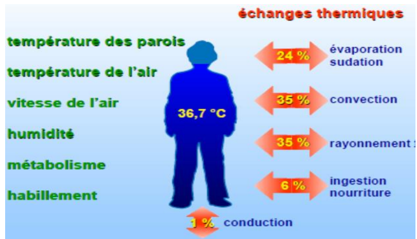
Figure 150: Les pertes thermiques dépendent de six paramètres physiques. Source : traité d'architecture et d'urbanisme bioclimatique.
