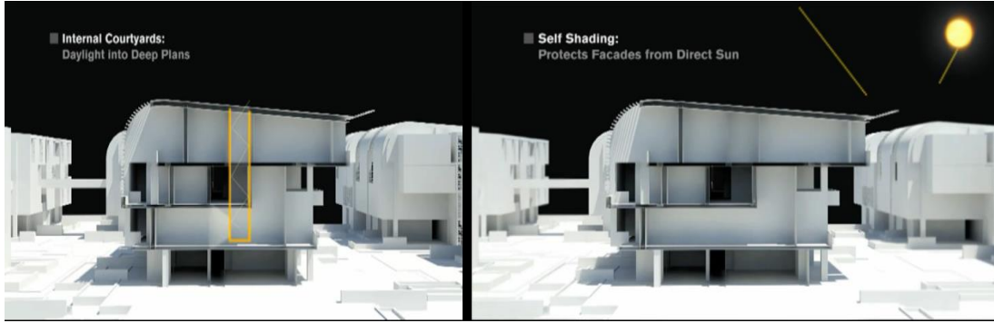
الصورة رقم (7) – توضح كيفية التعامل مع الاشعة الشمسية
