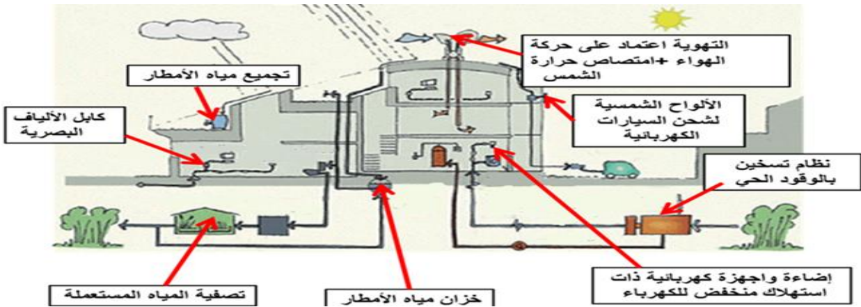
الصورة رقم (33) – توضح مخطط التهوية والتدفئة ودورة تخزين واستعمال مياه الأمطار والدائرة الكهربائية في إحدى المساكن المصدر: بحث حول الحي الايكولوجي من إعداد الطلبة بوزارة نسرين و بوعبيدي إيمان و بوعيشة سليمة الفوج 1. 2015/2014
