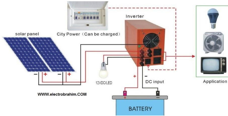
الصورة رقم (116) – توضح إستعمال الطاقة الشمسية بواسطة الألواح الشمسية
