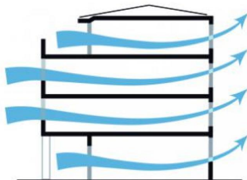
Figure n°04 : ventilation traversante Source : www.guidibatimentdurable.fr
