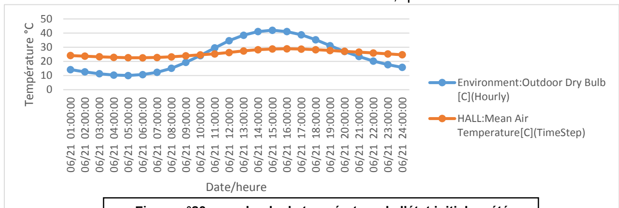
Figure n°20 : graphe de de température de l'état initial en été source : auteur
