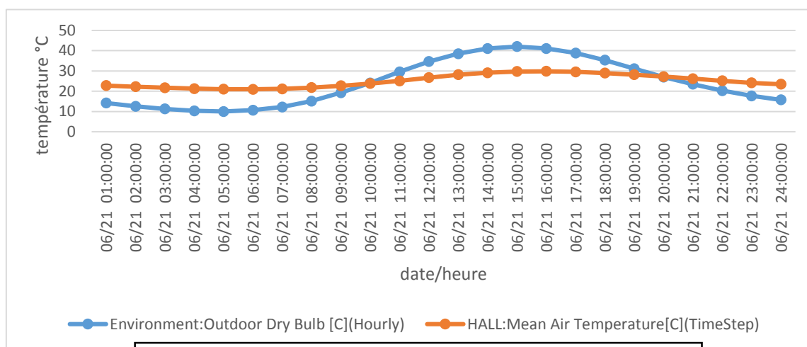
Figure n°22 : graphe de température à l'état corrigé été source : auteur
