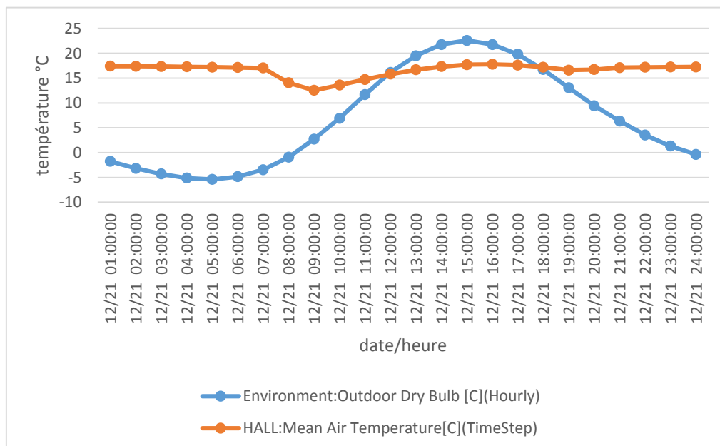
Figure n°26 : graphe de température à l'état corrigé hiver source : auteur
