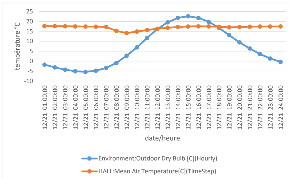
Figure n°24 : graphe de température de l'état initial en hiver source : auteur
