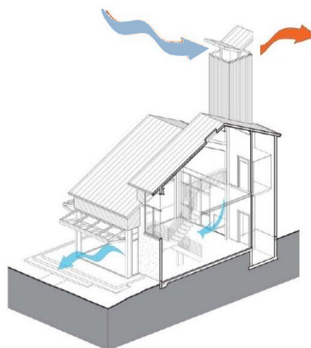
Figure n°11 : principe de fonctionnement de la tour à vent source : http://francouize.free.fr/
