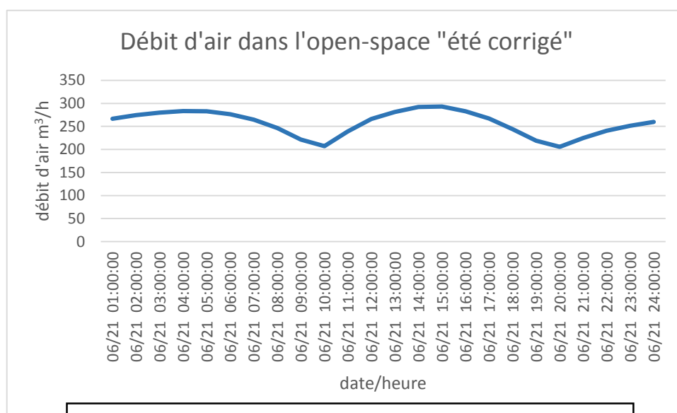
Figure n°21 : graphe de débit d'air à l'état corrigé été source : auteur
