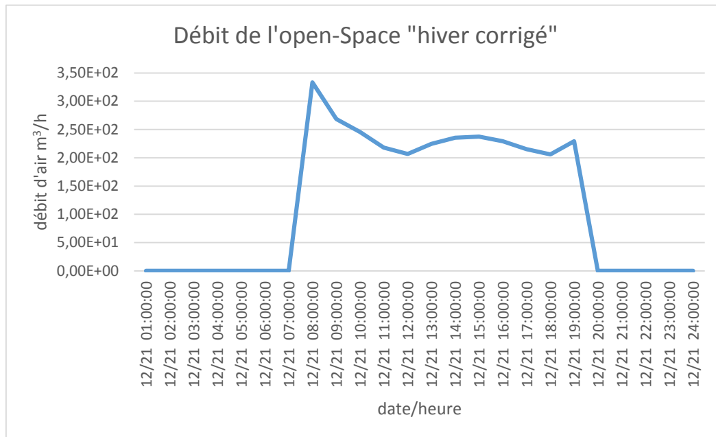
Figure n°25 : graphe de débit d'air à l'état corrigé hiver source : auteur
