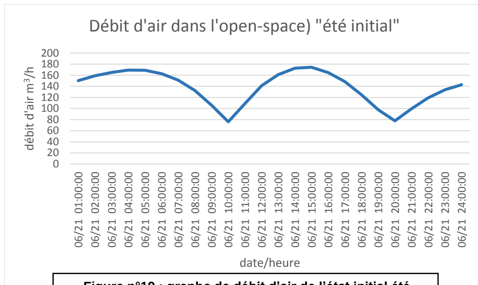
Figure n°19 : graphe de débit d'air de l'état initial été source : auteur
