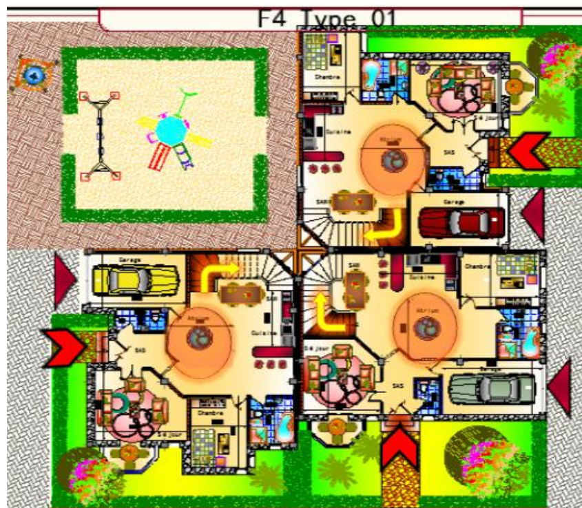
Figure IV.38 : plan de RDC du F4 type 01. Source : Auteur
