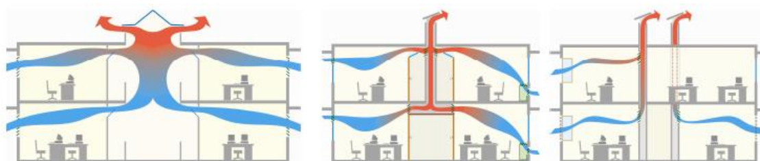
Figure n°06 : ventilation par tirage thermique Source : http://app.bruxellesenvironnement.be/
