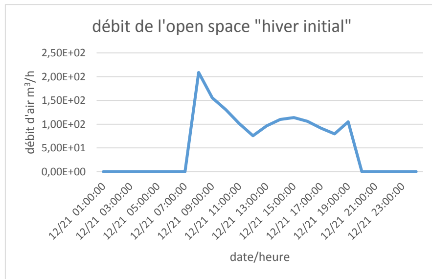
Figure n°23 : graphe de débit d'air de l'état initial en hiver source : auteur
