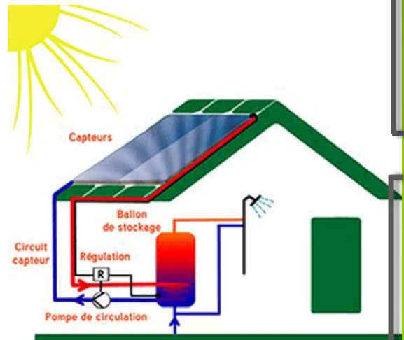
Figure III.6 : le principe de fonctionnement de Panneau solaire thermique source : www.college.lutterbach.free.fr
