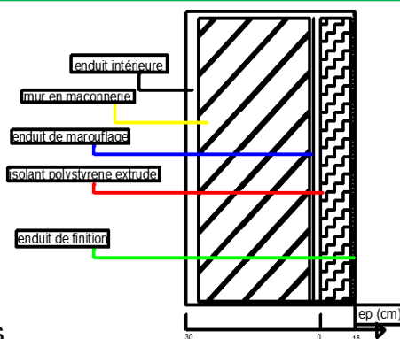
Figure 86 les différentes couches de l'isolation par extérieure
