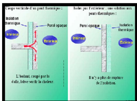
Figure 84 : isolation par l'extérieur
